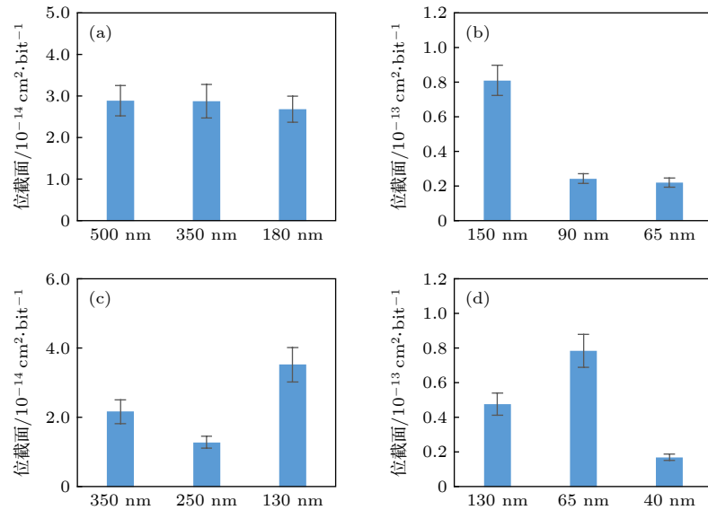
图6 同一厂商系列不同特征尺寸SRAM器件SEU截面对比 (a) HITECHI/RENESAS HM系列SRAM; (b) Cypress CY1318系列SRAM; (c) Cypress CY62126系列SRAM; (d) ISSI IS6X系列SRAM
