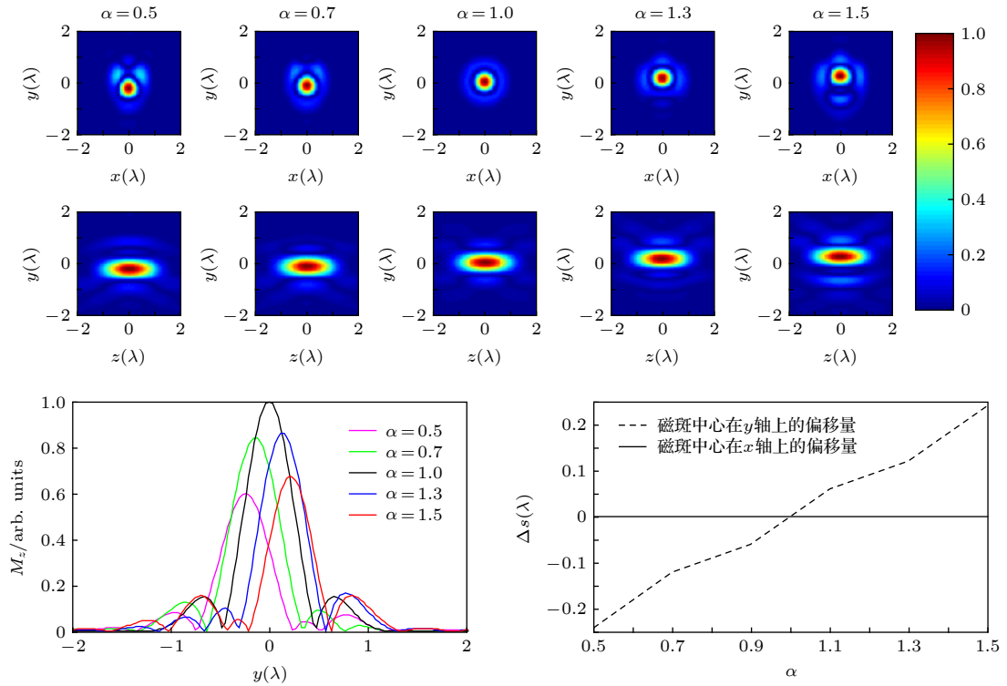
图 3 不同 \alpha 情况下磁化场强度分布 ( x - y 平面和 y - z 平面)、 z=0 截面强度及其峰值位置偏移图
