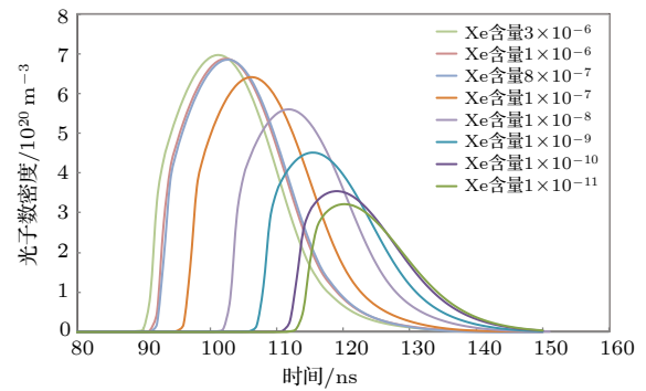
图 10 不同 Xe 含量光子数密度分布情况
