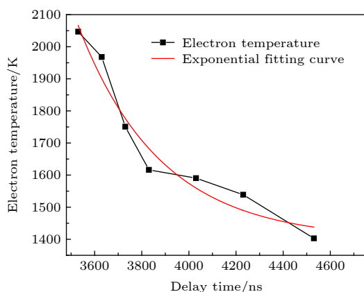
图 6 \text{SF}_6 等离子体电子温度随时间的演化过程
