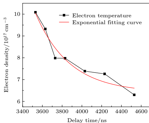
图 7 \text{SF}_6 等离子体电子密度随时间的演化过程
