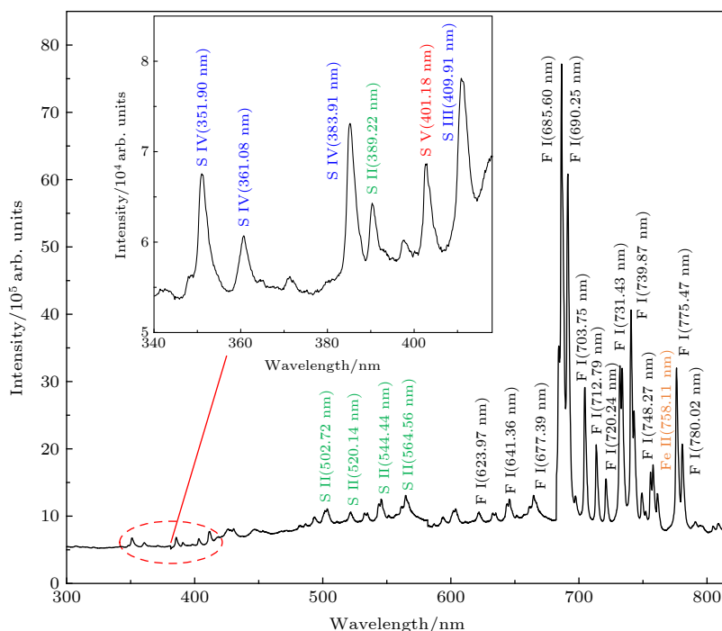
图 2 飞秒激光引导高压放电下的 \text{SF}_6 等离子体光谱图
