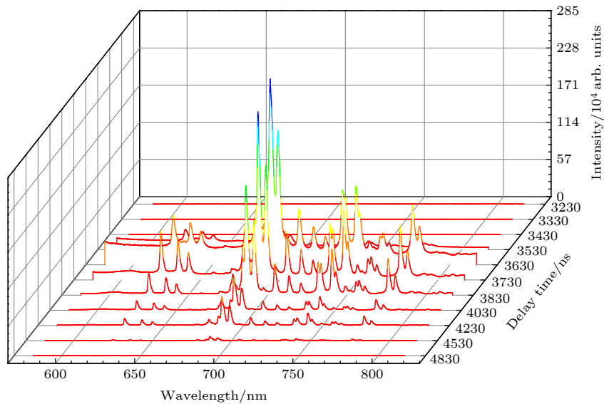
图 3 \text{SF}_6 等离子体时间分辨光谱
