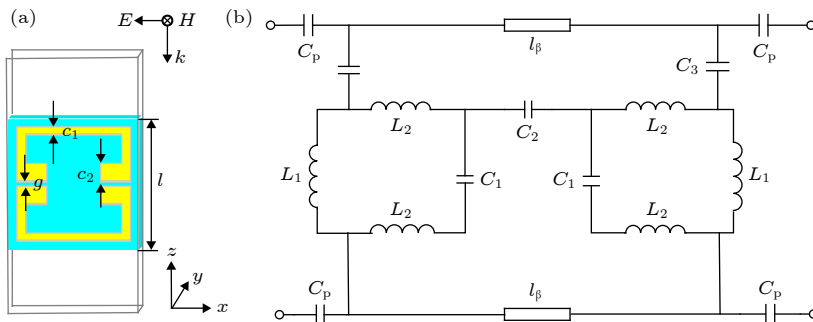
图 4 带阻 FSS (a) 单元设计; (b) 等效电路
