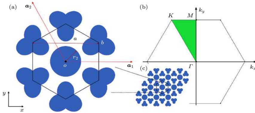
图 1 (a) 正六边形表示晶格的元胞, 其中 a_1, a_2 是晶格基矢. 在六边形顶点的蓝色“花瓣”形结构与位于中心的圆形结构表示位于空气中的硬质散射体; (b) 晶格的最简布里渊区 \Gamma - M - K ; (c) 晶格结构的示意图
