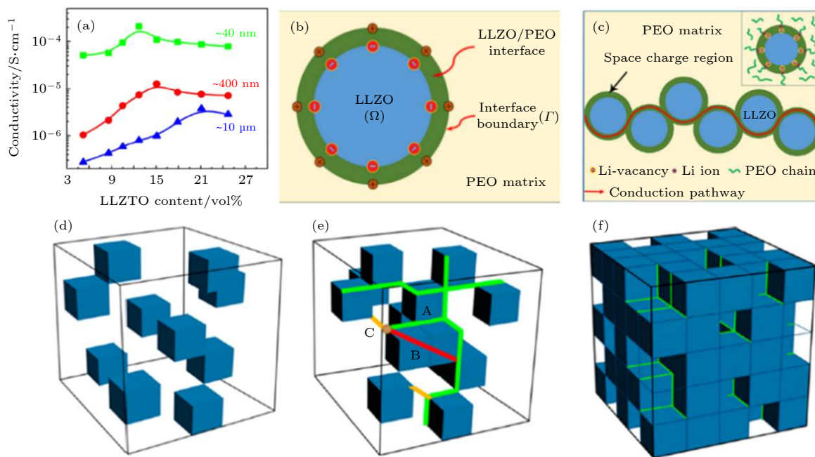
图 2 (a) 不同尺寸的锂镧锆氧 (LLZTO) 颗粒与聚环氧乙烷 (PEO) 制备复合电解质的室温离子电导率与 LLZTO 添加量的关系 [23] ; (b) LLZO-PEO 复合电解质内部界面结构示意图; (c) LLZO 与 PEO 界面的空间电荷层连接成快速离子传输通道的示意图; LLZO-PEO 复合电解质内形成渗流通道的过程: LLZO 添加量小于渗流阈值 (d); 到达渗流阈值 (e) 和超过渗流阈值 (f) 的示意图 [24]
