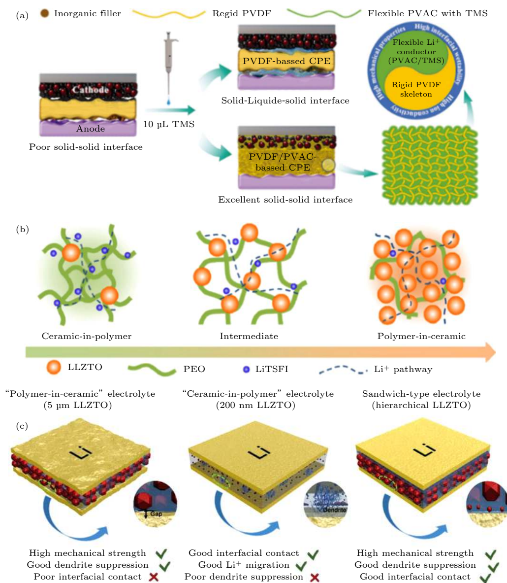
图 4 (a) “刚柔并济”的有机无机复合电解质膜的构建思路 [32] ; (b) “ceramic-in-polymer” (CIP) 和 “polymer-in-ceramic” (PIC) 复合电解质膜的结构示意图 [33] ; (c) 以 CIP 为外层、以 PIC 为内层的“外柔内刚”分级复合电解质膜 [34]
