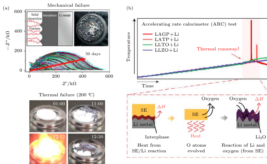
图 10 (a) NASICON 型氧化物固体电解质 LAGP 陶瓷片与金属锂的热稳定性研究 [61] ; (b) 采用加速量热仪研究 LAGP, LATP, LLTO 与 LLZO 四种氧化物固体电解质与金属锂接触时的热稳定性 [62]
