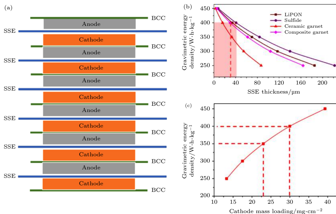
图 13 (a) 固体电解质 (solid state electrolyte, SSE) 与固态正负极以及双极性集流体 (bipolar current collector, BCC) 组成双极性电池结构的固态电池示意图; (b) 基于双极性电池结构, 四种固体电解质 (LiPON、硫化物、LLZO 陶瓷电解质与 LLZO 复合电解质) 厚度与质量能量密度的关系; (c) 固态复合正极的载量与质量能量密度的关系 [64] .
