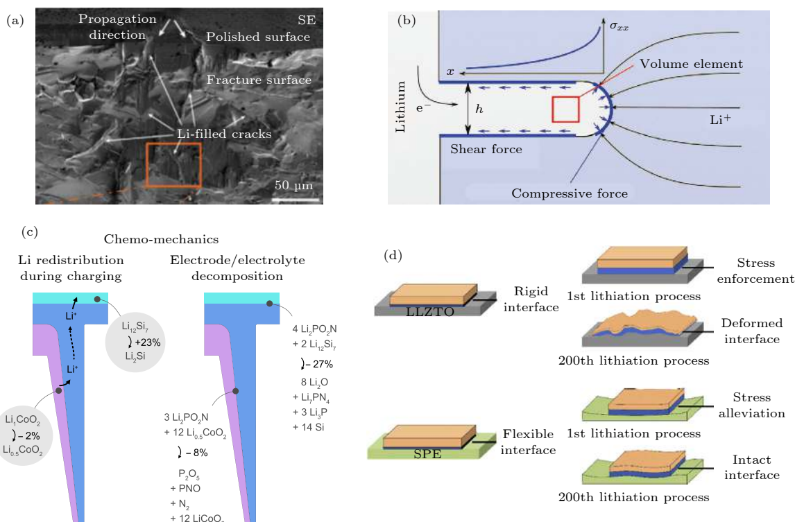
图 9 (a) 锂贯穿 LLZO 陶瓷电解质的微观形态分析 [57] ; (b) LLZO/Li 负极界面应力累积程度的简化模型 [58] ; (c) 硅负极/固体电解质界面应力应变产生的化学-力学耦合机制 [59] ; (d) 柔性复合固态电解质缓解硅负极产生的应力应变问题 [60]
