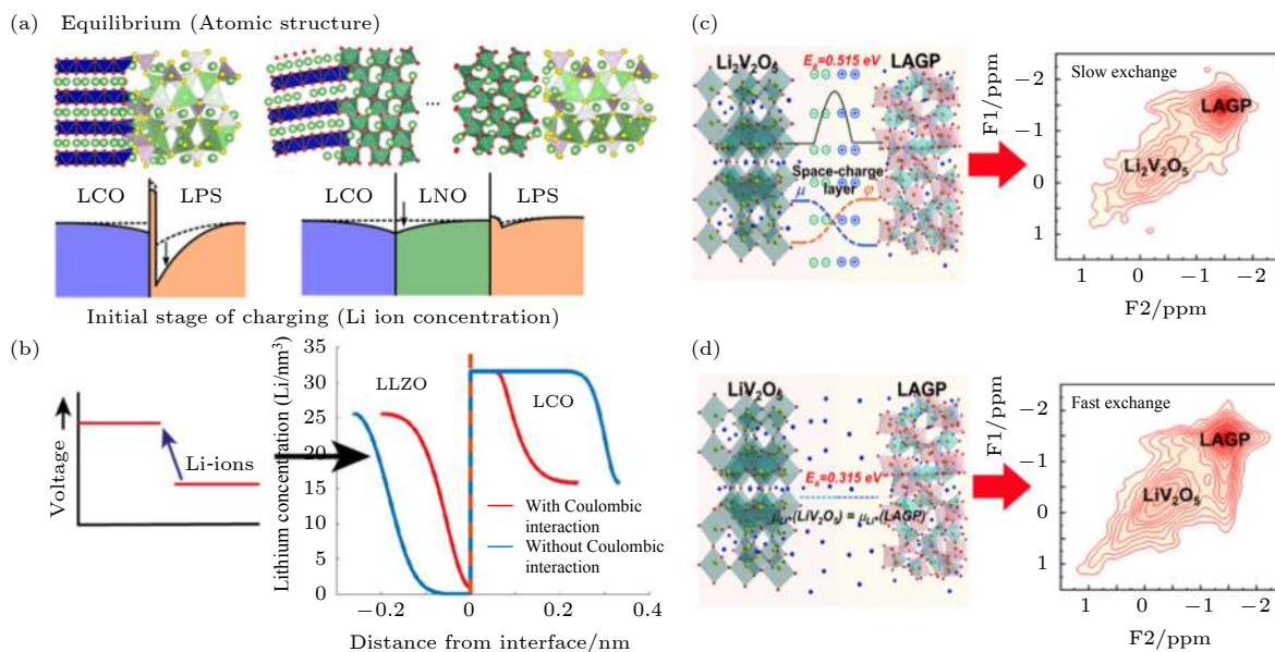
图 6 (a) 硫化物电解质/氧化物正极材料界面 [44] ; (b) 氧化物固体电解质/氧化物正极材料界面的空间电荷层示意图 [45] ; (c) LiV 2 O 5 /LAGP 和 (d) Li 2 V 2 O 5 /LAGP 界面的空间电荷层与对应的固态核磁共振交换谱 [46]
