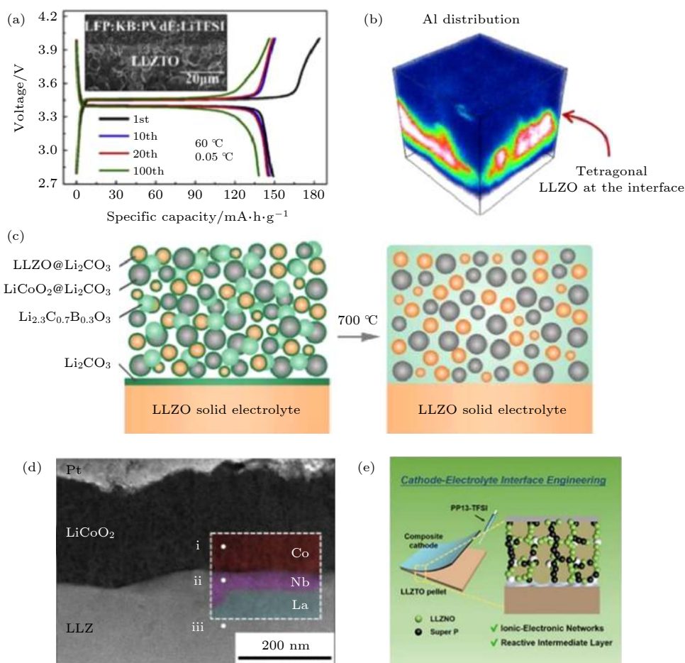
图 5 (a) 采用传统电极涂布法制备的固态复合正极及其充放电曲线 [12] ; (b) LLZO/LiCoO 2 界面发生元素互扩散形成四方相 LLZO [13] ; (c) 引入低熔点助烧剂 Li 2.3 C 0.7 B 0.3 O 3 (LCBO) 后, LLZO 与 LiCoO 2 形成离子导电的稳定界面 [36] ; (d) 金属 Nb 中间层有效抑制 LLZO 与 LiCoO 2 间的元素互扩散 [37] ; (e) 结合表面包覆和原位电化学法在固态正极中形成离子电子共导电网络 [38]
