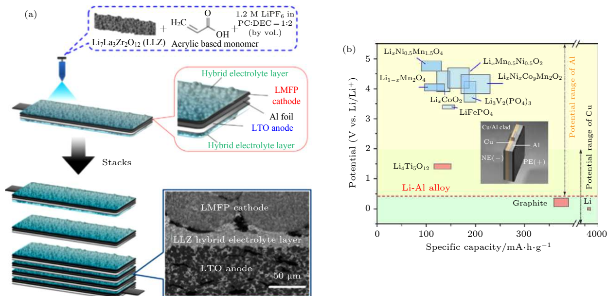
图 12 (a) 由 LMFP 正极、LLZO 基混合电解质层和 LTO 负极组成的双极性准固态电池的截面示意图和截面 SEM 图像 [69] ; (b) 集流体 Al 和 Cu 的稳定电位范围以及 Cu/Al 双极性集流体的示意图 [65,69]
