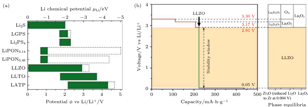
图 1 (a) 常见氧化物与硫化物固体电解质的热力学稳定窗口 [17] ; (b) \text{Li}_7\text{La}_3\text{Zr}_2\text{O}_{12} 的热力学稳定窗口第一性原理计算结果 [18]
