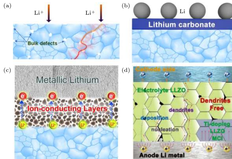
图 8 (a) 低致密度且有晶格缺陷的 LLZO 陶瓷电解质示意图 [52] ; (b) 表面碳酸锂等污染物对 LLZO 陶瓷亲锂性的影响; (c) 理想的纯离子导体中间层有效抑制金属锂贯穿, (d) 在 LLZO 陶瓷电解质近锂侧掺 Ti, 在陶瓷本体部分形成混合离子电子导电界面起到均匀化电场、阻挡电子注入和抑制锂成核等作用 [53]
