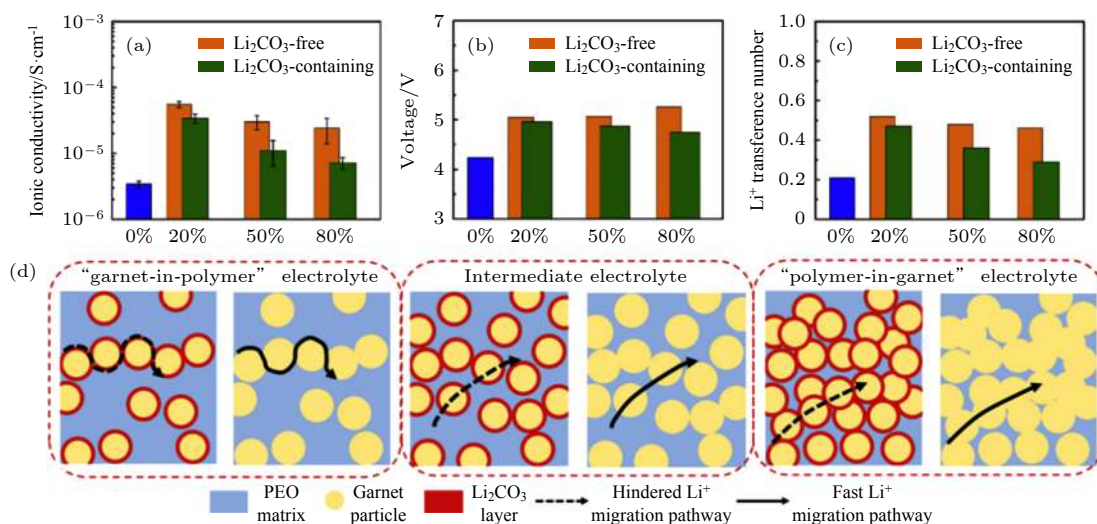
图 3 有无 \text{Li}_2\text{CO}_3 的 LLZO 与 PEO 形成复合电解质膜的 (a) 离子电导率; (b) 电化学窗口; (c) 锂离子迁移数的对比; (d) \text{Li}_2\text{CO}_3 对复合电解质中锂离子传输途径影响的示意图 [26]
