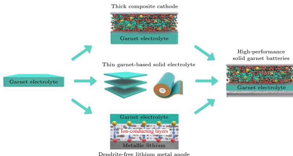
图 11 能量密度大于 400 Wh/kg 的石榴石型固态电池开发策略 [64]
