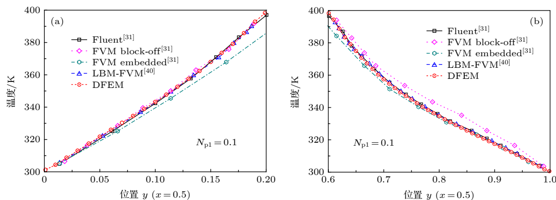
图 6 不同数值方法得到的半圆介质对称线上温度分布 (a) y = [0.0, 0.2] ; (b) y = [0.6, 1.0]
