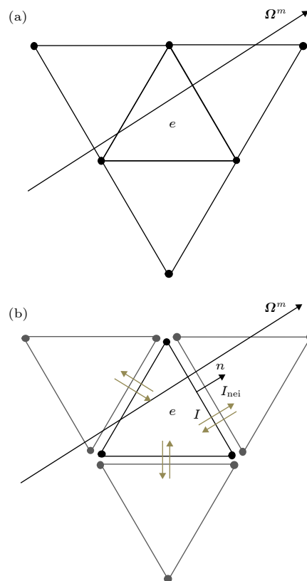
图 1 (a) 空间网格; (b) 相邻单元间数值通量示意图
