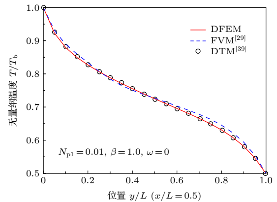
图4 不同数值方法得到的方形介质对称线上的无量纲温度对比
