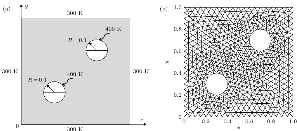
图 10 内含两个圆形热边界的矩形介质 (a) 结构示意图; (b) 网格划分
