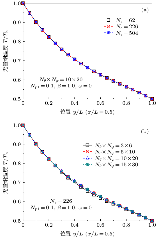
图2 方形介质对称线 x/L = 0.5 上无量纲温度 T/T_b 分布 (a) 不同空间网格划分; (b) 不同角度划分
