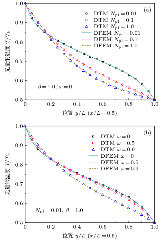
图3 方形介质对称线 x/L = 0.5 上无量纲温度的 DFEM 结果和 DTM 结果对比 (a) 不同普朗克数; (b) 不同散射反照率
