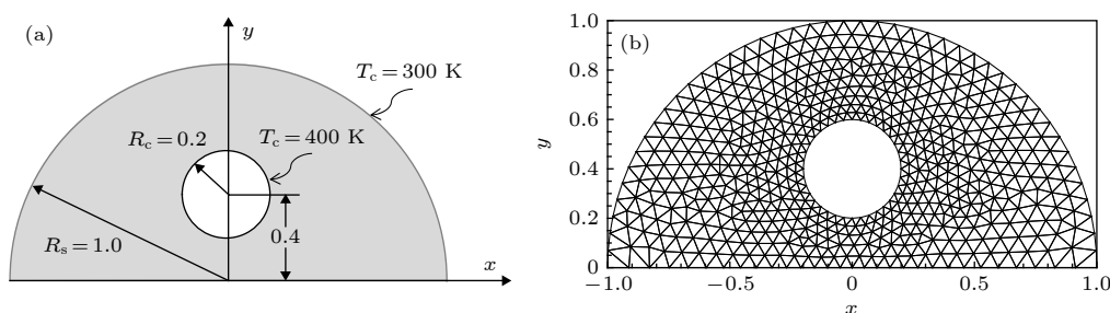
图 5 内含圆形热壁面的半圆形介质 (a) 结构示意图; (b) 网格划分
