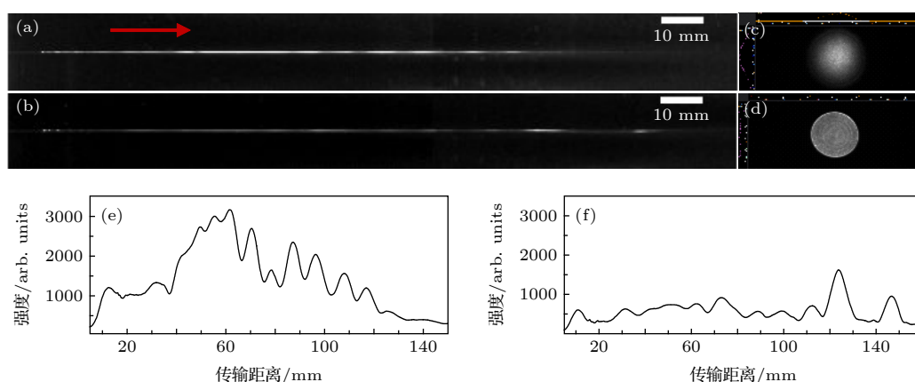
图2 飞秒高斯激光((a), (c), (e))和平顶激光((b), (d), (f))的初始光斑((c), (d))及其在熔融石英中成丝的荧光图像((a), (b)),以及成丝轴线上荧光强度((e), (f))随传输距离的演化.实验中使用的激光脉冲能量均为 672 \mu\text{J} .图中箭头方向表示激光传输方向
