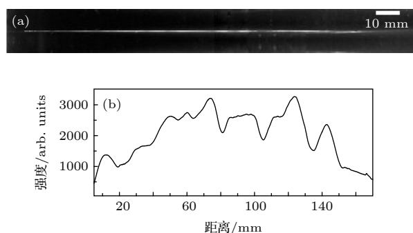
图 3 入射能量为 1.319 mJ 的平顶激光经圆锥透镜在熔融石英中形成的细丝荧光图像 (a) 及其光轴上的强度随传输距离的演化 (b)
