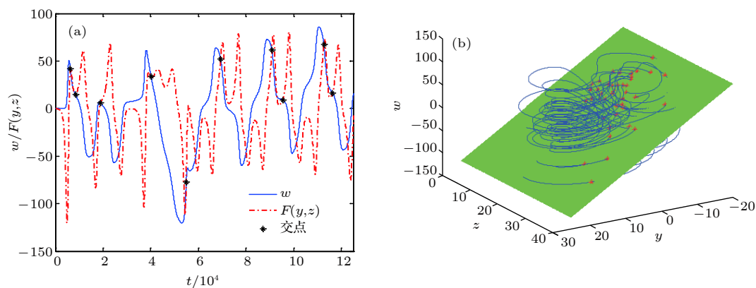
图 12 x = 0 时的实验结果 (a) 波形; (b) 相图
