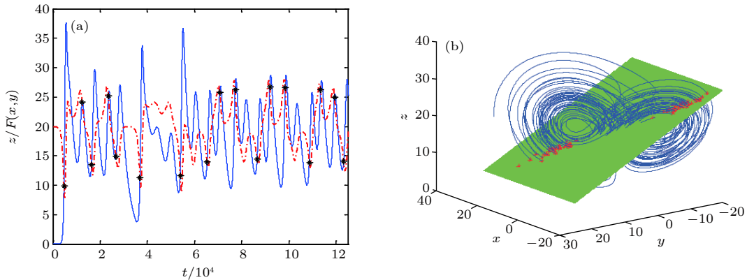
图 9 w = 0 时的实验结果 (a) 波形; (b) 相图
