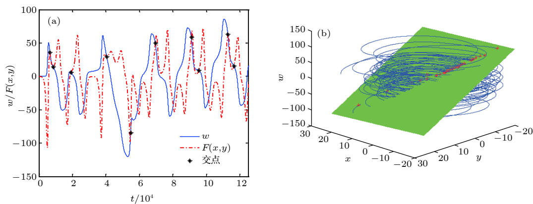
图 10 z = 0 时的实验结果 (a) 波形; (b) 相图
