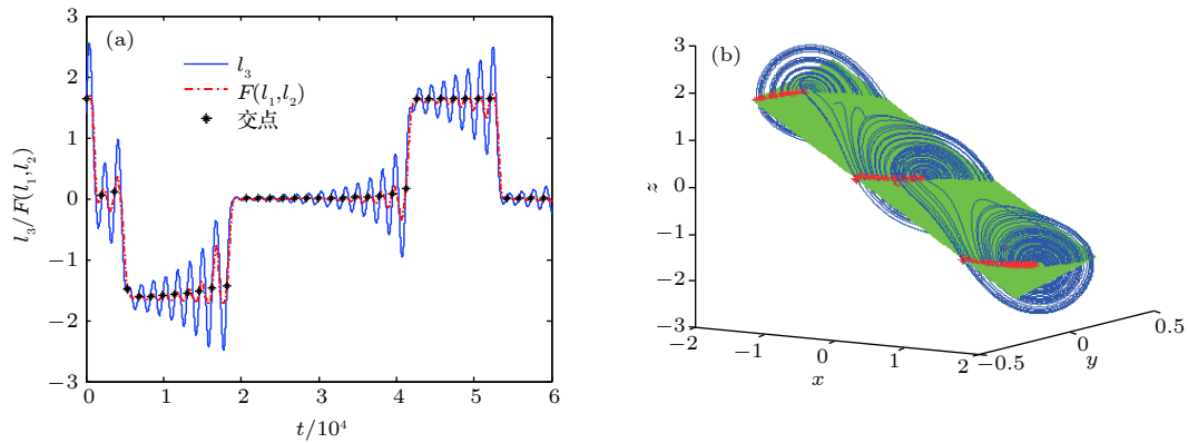
图 8 平面二的实验结果 (a) 波形; (b) 相图
