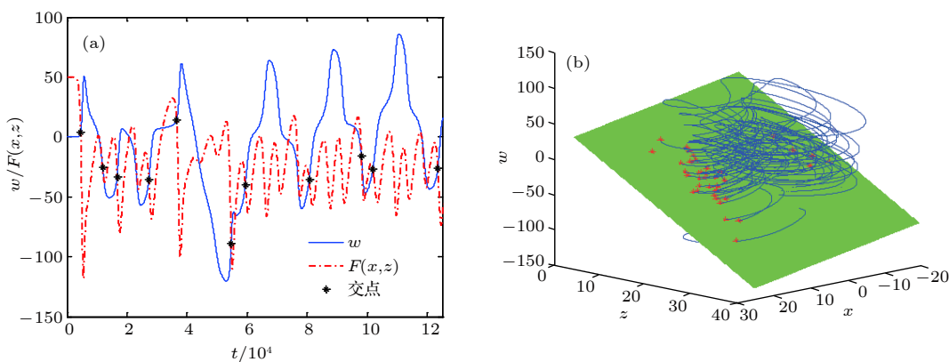
图 11 y = 0 时的实验结果 (a) 波形; (b) 相图
