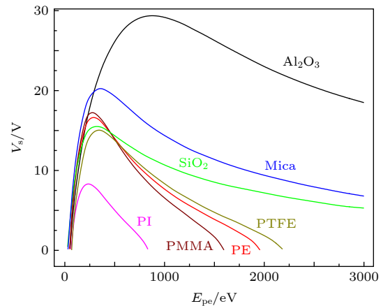
图 4 稳态表面电位与入射电子能量的关系
