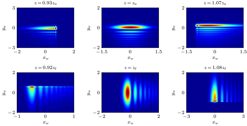
图 2 金红石晶体时不同传输距离处的光束强度分布, 其他参数分别为 N_w = 1 , a = b = 0.1 , \delta = 1
