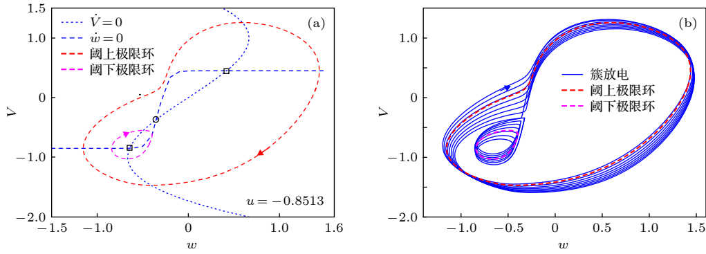
图2 改进FHN模型的快子系统和全系统在相平面 (w, V) 的动力学行为 (a) u = -0.8513 时快子系统的阈上极限环(红色虚线)和阈下极限环(洋红色虚线), 箭头表示轨线运行方向, \dot{V} 的零值线(蓝色点线)和 \dot{w} 的零值线(蓝色虚线), “□”表示不稳定焦点, “○”表示鞍点; (b) 全系统周期8簇放电的轨线在相平面 (w, V) 的投影(蓝色实线, 箭头为运行方向)与图(a)中阈上(红色虚线)和阈下极限环(洋红色虚线)的叠加
