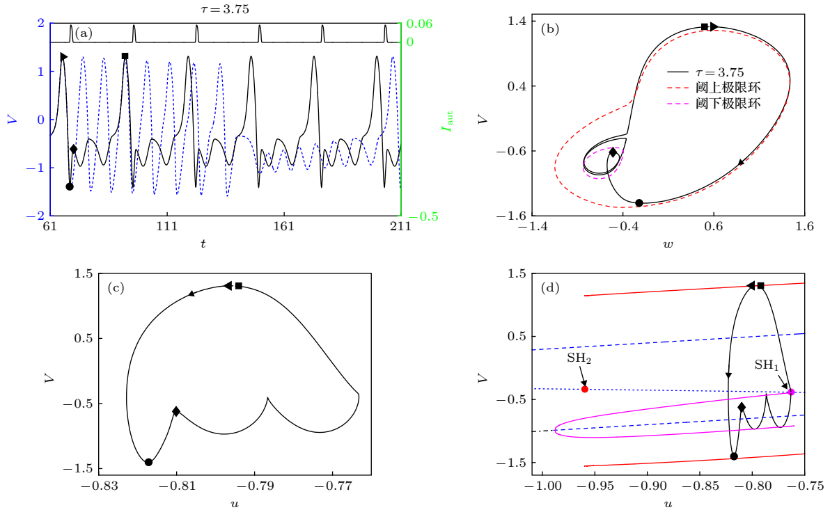
图4 具有兴奋性自突触的改进FHN模型在 g = 0.02 和 \tau = 3.75 时的新放电模式及其慢变量分离 (a) 周期8簇(蓝色点线)在兴奋性自突触电流(上黑色实线)作用下诱导出新的放电模式(下黑色实线); (b) 自突触的作用下新模式(►到■时段)在相平面( w, V )的投影, 轨线在相位●从阈上极限环(红色虚线)跃迁到阈下极限环(洋红色虚线); (c) 新放电模式(►到■时段)在相平面( u, V )的投影; (d) 图(c)与快子系统分岔图1(b)的叠加
