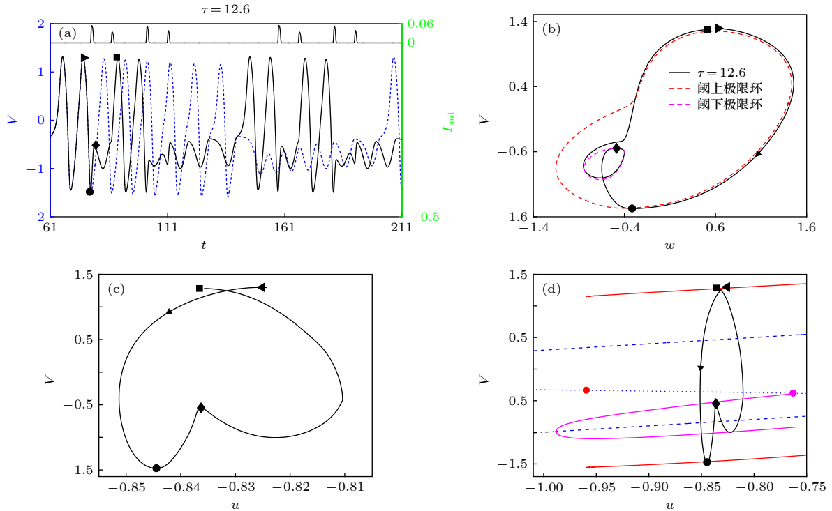
图 5 具有兴奋性自突触的改进 FHN 模型在 g = 0.02 和 \tau = 12.6 时的新放电模式及其快慢变量分离 (a) 周期 8 簇 (蓝色点线) 在兴奋性自突触 (上黑色实线) 作用下诱导出新放电模式 (下黑色实线); (b) 自突触的作用下新模式 (►到■时段) 在相平面 ( w, V ) 的投影, 轨线在相位●从阈上极限环 (红色虚线) 跃迁到阈下极限环 (洋红色虚线); (c) 新放电模式 (►到■时段) 在相平面 ( u, V ) 的投影; (d) 图 (c) 与快子系统分岔图 1(b) 的叠加
