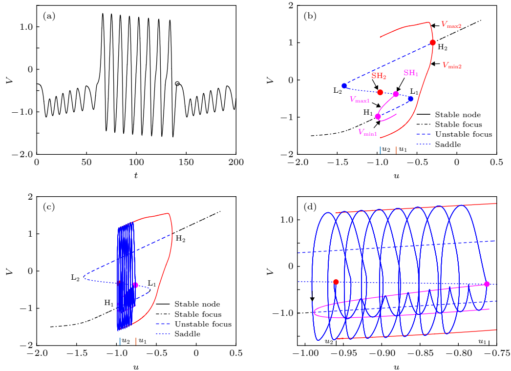
图1 改进FHN模型簇放电模式及其快慢变量分离 (a) 周期8簇 (圆圈对应 V = -0.3396 , t = 141.15 ); (b) 快子系统的分岔, 其中黑色实线、黑色虚线、蓝色点线和蓝色虚线分别表示稳定结点、稳定焦点、鞍点和不稳定焦点; L_1 和 L_2 为两个鞍结分岔点、 H_1 和 H_2 为两个Hopf分岔点; 从 H_1 开始的上下两个洋红色实线分别表示阈下稳定极限环的最大值与最小值, SH_1 为鞍同宿轨分岔点, 对应 u_1 = -0.760022 ; 从 H_2 开始的上、下两个红色实线分别表示阈上稳定极限环的最大值与最小值, SH_2 为鞍同宿轨分岔点, 对应 u_2 = -0.959267 ; (c) 图(b)与周期8簇放电轨线 (蓝色实线) 的叠加; (d) 图(c)的局部放大
