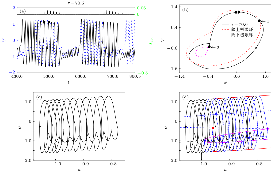
图 7 具有兴奋性自突触的改进 FHN 模型在 g = 0.02 和 \tau = 70.6 时的新放电模式及其快慢变量分离 (a) 周期 8 簇 (蓝色点线) 在兴奋性自突触 (上黑色实线) 作用下诱导出新的放电模式 (下黑色实线); (b) 自突触的作用下新模式 (图 (a) 中 \blacktriangleright 到 \blacksquare 时段) 在相平面 ( w, V ) 的投影; 第 1 个兴奋脉冲作用在相位 \bullet 1 , 在放电峰上没有引起放电峰大的变化; 第 2 个兴奋脉冲作用在相位 \bullet 2 , 使本来应该产生的阈下振荡变成阈上放电; (c) 新放电模式在相平面 ( u, V ) 的投影; (d) 图 (c) 和原放电轨线 (蓝虚线) 及快子系统分岔图 1(b) 的叠加
