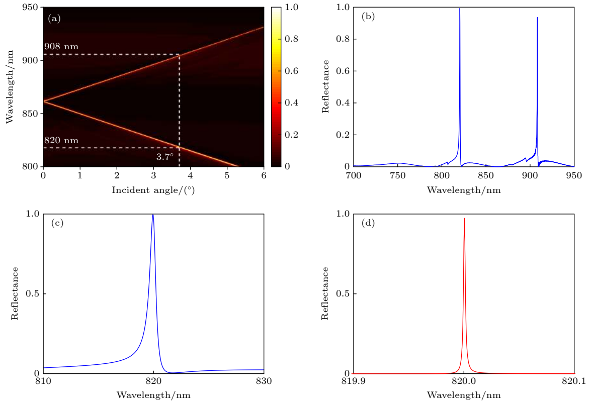
图 2 (a) TE 偏振下多孔二氧化硅结构的反射谱随入射角和波长的变化曲线; (b) 3.7°入射角下多孔二氧化硅结构的反射谱; (c) 3.7°入射角下多孔二氧化硅结构的 820 nm 共振峰; (d) 21.3°入射角下 SU-8 结构的 820 nm 共振峰
