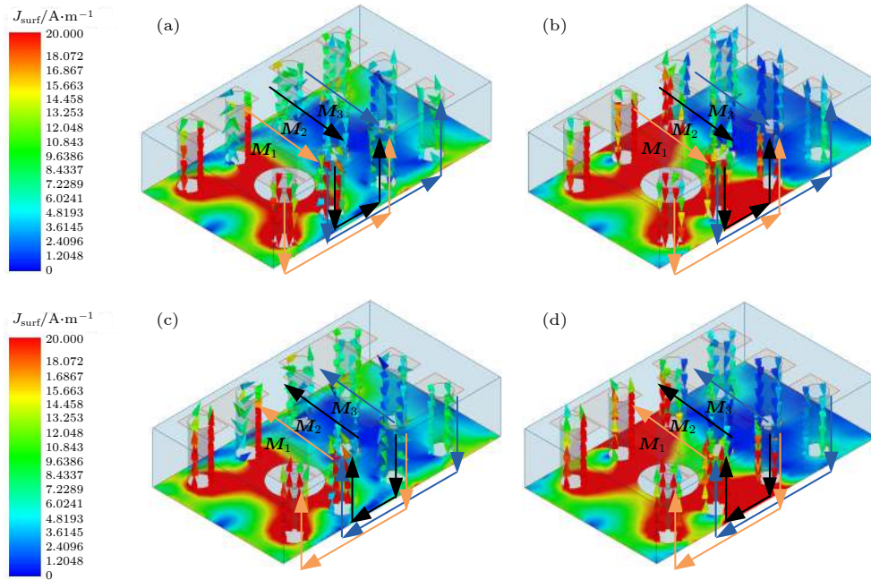
图 4 10 GHz 处电流分布图 (a) 0°; (b) 90°; (c) 180°; (d) 270°
