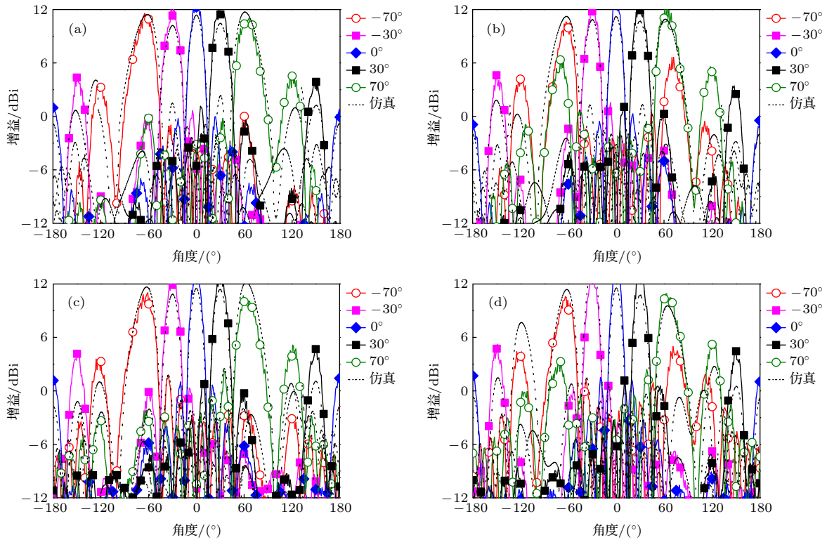
图 10 E面阵列实测扫描方向图 (a) 9 GHz; (b) 10 GHz; (c) 11 GHz; (d) 12 GHz
