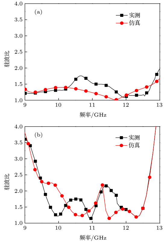
图 9 阵列中心单元实测有源驻波比 (a) E面阵列; (b) H面阵列
