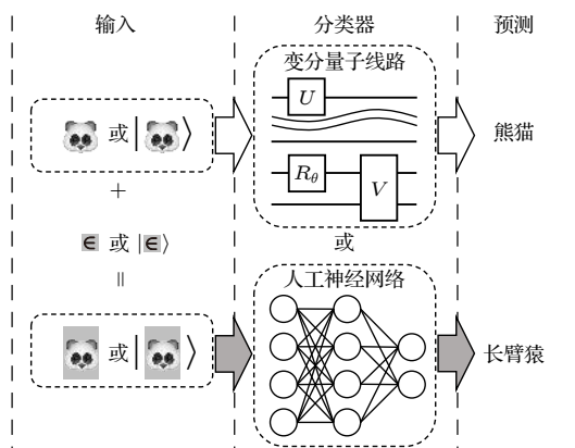
图 1 量子与经典对抗学习示意图 输入的原始熊猫图像样本可以编码为经典或量子数据, 分类器 (包含变分子线路或人工神经网络) 能够以非常高的准确率识别出熊猫; 但添加少量精心制作的噪声后, 同一分类器将以非常高的置信度把轻微修改过的熊猫图像错误分类为长臂猿
