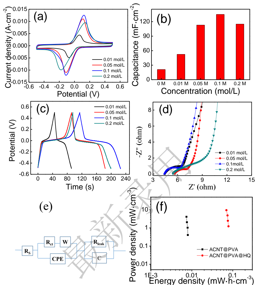
图3 不同浓度下 ACNT@PVA@HQ 器件的电化学性能测试 (a)相同扫速(20 mV/s)下不同 HQ 添加量的器件 CV 对比图; (b)器件比容量随 HQ 浓度变化图; (c)相同电流密度(1.23 mA·cm -2 )下的 GCD 曲线对比图; (d)交流阻抗谱对比图; (e)等效电路拟合模型图; (f) ACNT@PVA@HQ(0.1M)器件与 ACNT@PVA 器件 Ragone 对比图
