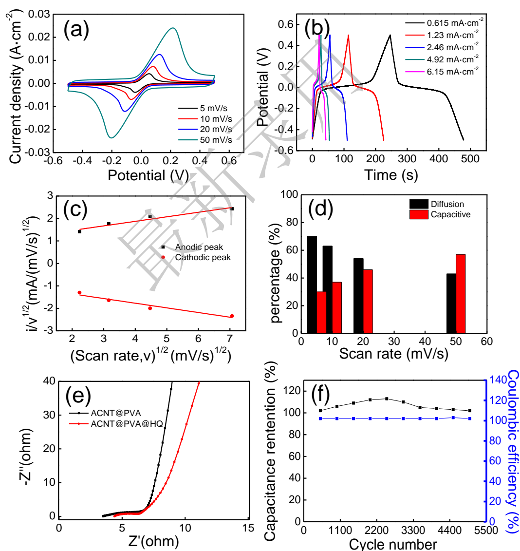
图 4 [HQ]=0.1 \text{ mol/L} 浓度下 ACNT@PVA@HQ 器件的电化学性能测试 (a)循环伏安曲线图 (5-50 mV/s); (b)不同电流密度( 0.615 \text{ mA}\cdot\text{cm}^{-2} - 6.15 \text{ mA}\cdot\text{cm}^{-2} )下的 GCD 曲线图; (c)峰电流与扫速的关系图; (d)容量贡献占比图; (e)交流阻抗谱图; (f)5000 次循环稳定性图
