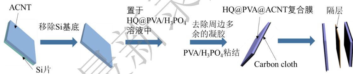
图 1 HQ@PVA@ACNT 氧化还原增强型固态超级电容器器件组装过程示意图
