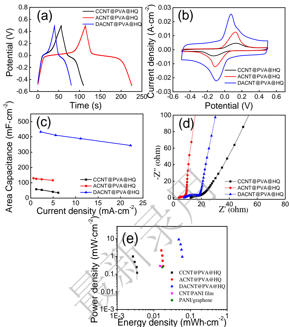
图 5 CCNT@PVA@HQ, ACNT@PVA@HQ 和 DACNT@PVA@HQ 器件的电化学测试 (a) 相同电流(1 mA)下的 GCD 对比图; (b) 20 mV/s 下的 CVs 对比图; (c) 面积比容量随电流密度变化图; (d) EIS 对比图; (e) 器件功率密度-能量密度对比图
