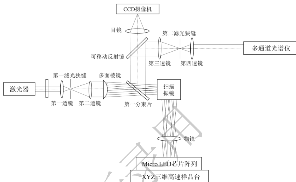
图 14 micro-LED 芯片共焦显微拉曼结合光致发光检测系统示意图 [146]
