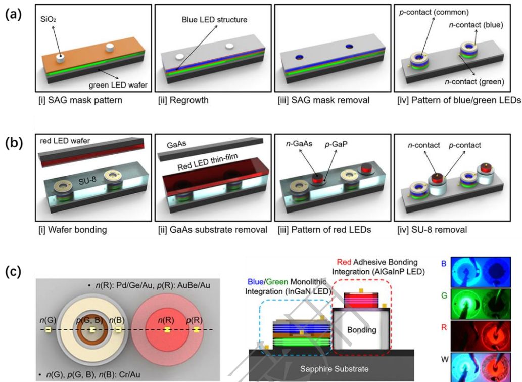
图 9 RGB LED 的制备过程示意图：(a)使用选择性区域生长制备蓝光和绿光双色 LED；(b)使用粘合剂集成红光 LED 的过程；(c)最终器件的俯视图和横截面图，RGB LED 以蓝光、绿光、红光和白光模式(从上到下)依次显示的显微图像 [107]
