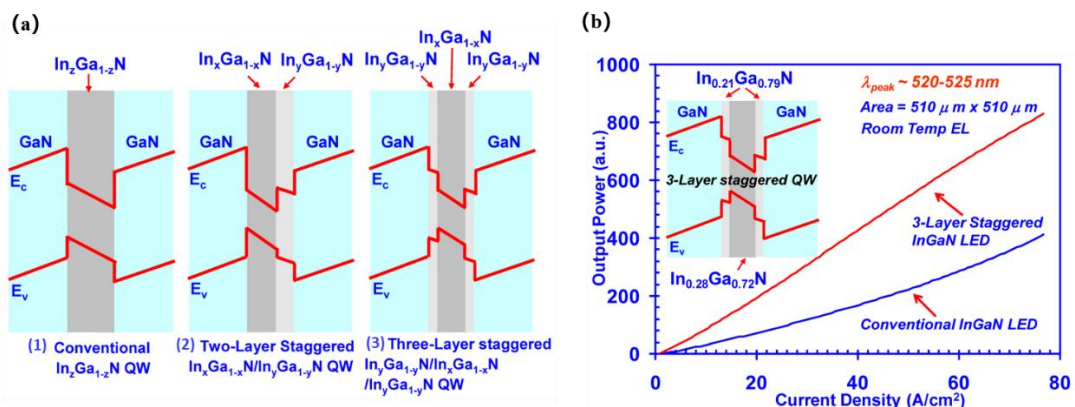
图 3 (a)常规的 In x Ga 1-x N-GaN 量子阱、两层交错的 In x Ga 1-x N/In y Ga 1-y N 量子阱和三层交错的 In y Ga 1-y N/In x Ga 1-x N/In y Ga 1-y N 量子阱的示意图；(b)基于常规 InGaN 量子阱和三层交错的 InGaN 量子阱的 LED 在波长 520-525 nm 范围内光输出功率与电流密度的关系，插图为
