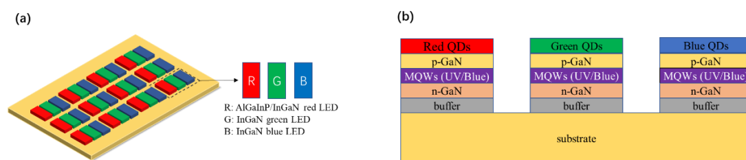
图 8 (a) 分立 RGB 排列法; (b) UV/Blue LED 激发量子点法
