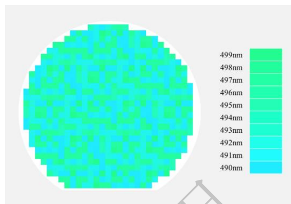
图 6 典型的 Micro-LED 发光波长在外延片上的分布
