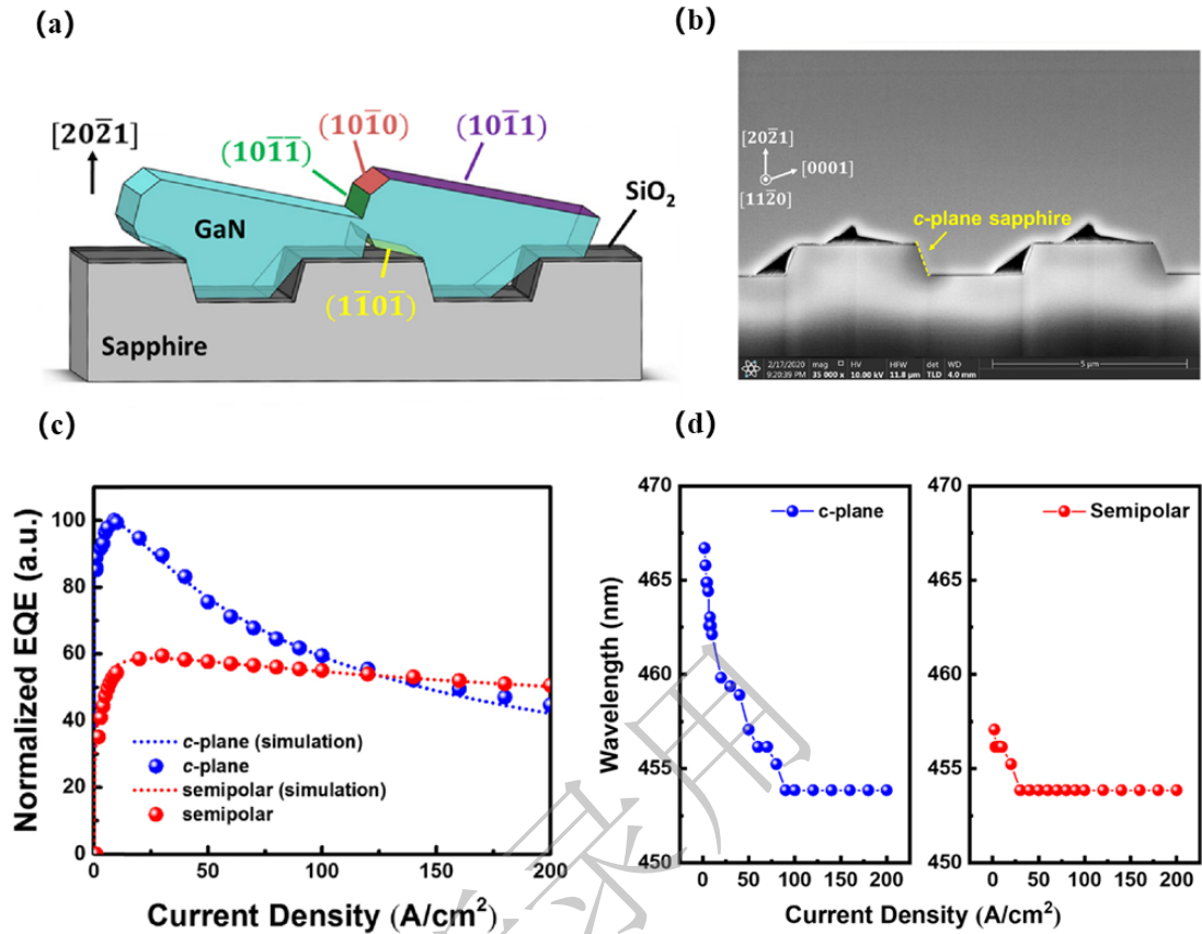
图 5 (a)在图形化蓝宝石衬底上生长的半极性 GaN 示意图；(b)通过取向控制外延在图形化蓝宝石衬底上生长的(20-21) GaN 截面的扫描电子显微镜图像；(c) c 面和半极性面 micro-LED 归一化 EQE 的实验数据和仿真曲线；(d)当电流密度在 1 至 200 \text{ A}/\text{cm}^2 范围内变化时 c 面和半极性面 micro-LED 的峰值波长 [86]
