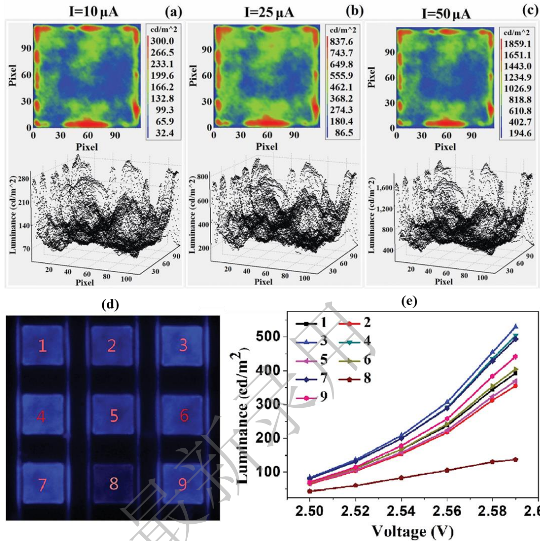
图 15 (a)~(c) 单个 micro-LED 芯片不同电流对应的亮度的伪彩色图和 3D 分布; (d) micro-LED 阵列中的部分芯片; (e) 这些芯片在不同电压下的平均亮度 [159]
