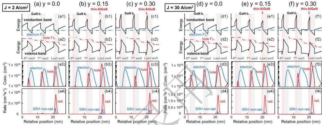
图 4 含有 \text{Al}_y\text{Ga}_{1-y}\text{N} 薄插入层的量子阱的能带图、载流子分布和复合速率 (a)和(d): 量子阱中 Al 组分摩尔系数 y=0 ; (b)和(e): 量子阱中 Al 组分摩尔系数 y=0.15 ; (c)和(f): 量子阱中 Al 组分摩尔系数 y=0.3 ; (a)~(c)和(d)~(f)的工作电流密度分别设定为 2 和 30\text{ A/cm}^2 [76]
