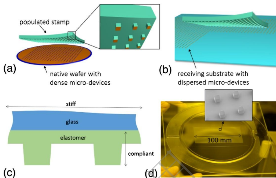
图 12 (a)转移印模从装有密集微器件的原晶圆上获取微器件阵列；(b)将分散的微器件转移到接收基板上；(c)转移印模的横截面示意图；(d)有效面积 100\ \text{mm}\times 50\ \text{mm} 的转移印模阵列照片，插图弹性印模表面的电子显微镜图像 [130]
