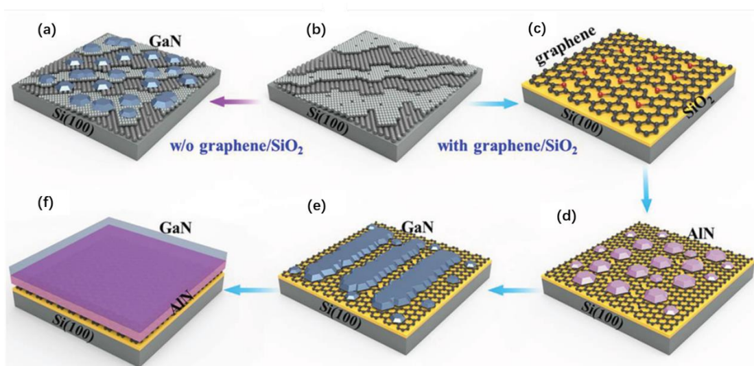
图 2 在具有和不具有单晶石墨烯/SiO 2 缓冲层的 Si(100)上分别生长单晶 GaN 薄膜的示意图 (a)在 Si(100)上直接生长 GaN/AlN,氮化物在两种不同取向的台面上成核; (b)Si(100)的表面结构; (c)NH 3 预处理后转移的石墨烯; (d)石墨烯上的 AlN 成核岛; (e)在 AlN 成核层上生长的
