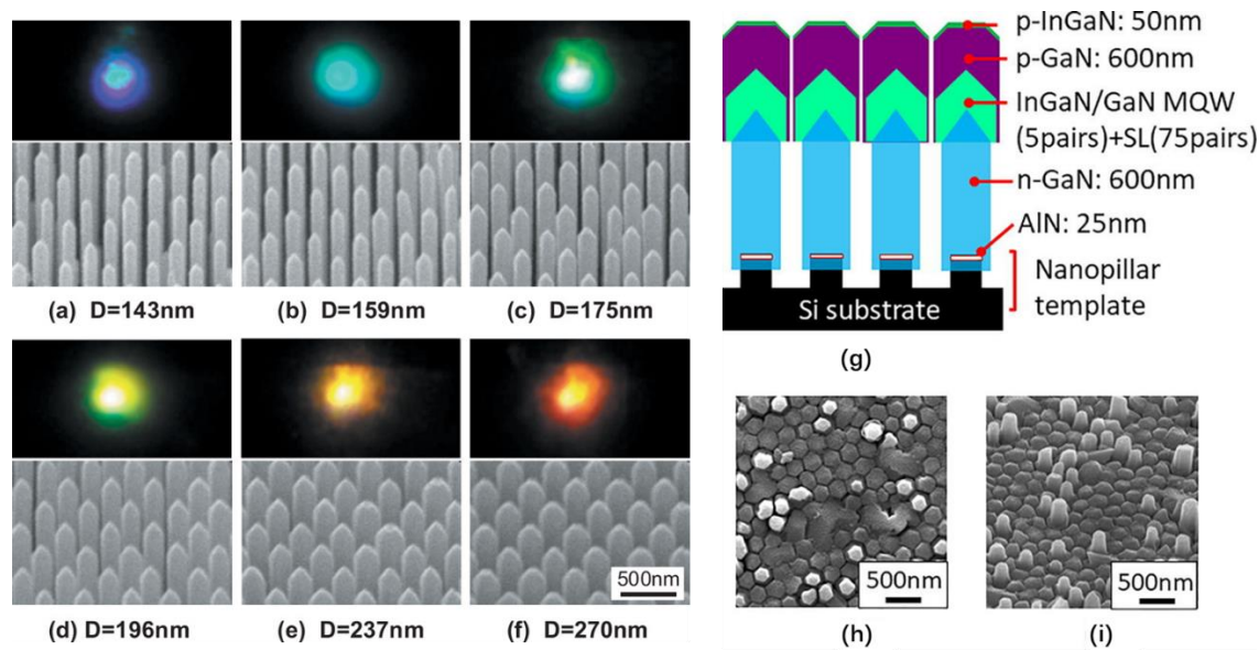
图 11 SEM 鸟瞰图和 He-Cd 激光器激发的不同直径 InGaN/GaN 纳米柱的发射图像：(a)143 nm; (b)159 nm; (c)175 nm; (d)196 nm; (e)237 nm; (f)270 nm [116] ；AlN/Si 纳米模板上的 InGaN 纳米柱 LED：(g)InGaN 纳米柱 LED 示意图；(h)纳米柱 LED 的 SEM 俯视图；(i)纳米柱 LED 的 SEM 鸟瞰图 [117]
