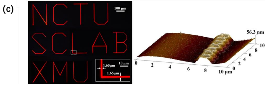
图 10 (a)基于量子点的全彩色显示 micro-LED 的制备流程 [10] ; (b)光刻胶模具的光学显微镜图像, 其尺寸为 35\ \mu\text{m}\times 35\ \mu\text{m} 、间距约为 40\ \mu\text{m} , 以及光刻胶模具的激光扫描仪显微镜图像, 其模板高度为 11.46\ \mu\text{m} [111] ; (c)荧光显微镜下使用最新的超微喷墨印刷技术在玻璃上用红色量子点印刷的图案 (插图描绘了最小线宽) 以及沉积的量子点的原子力显微镜图像 [17]
