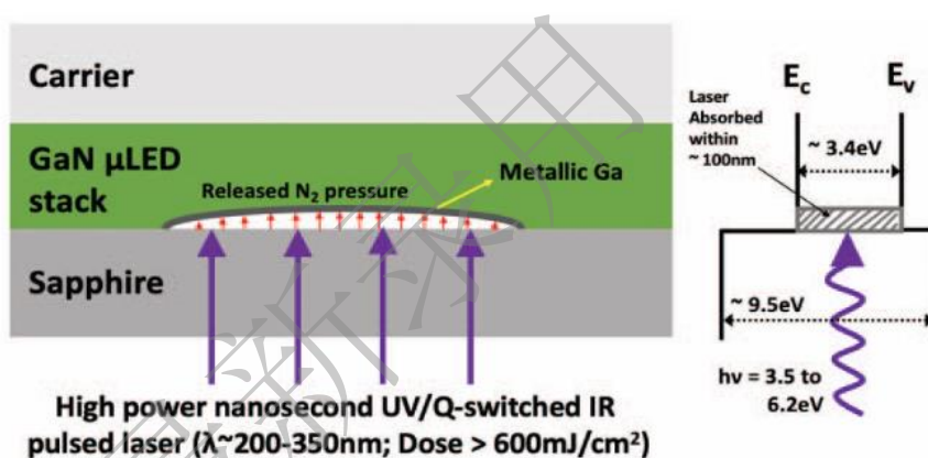
图 13 激光剥离工艺的示意图和氮化镓/蓝宝石界面的能带图 [139]
