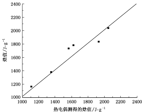
图5 热电偶与焓探针测量的焓值的比较
