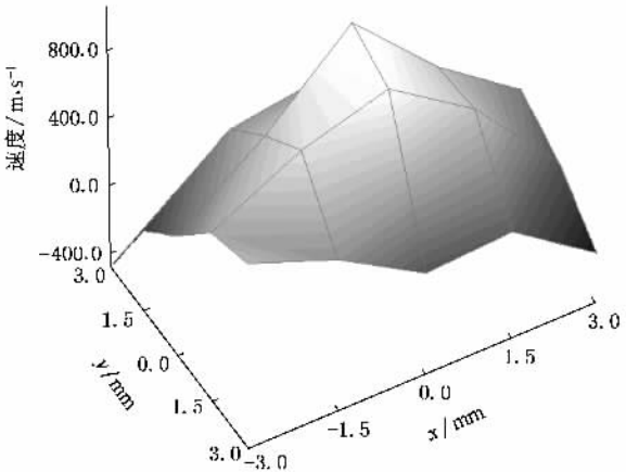
图 7 所测截面的速度分布
