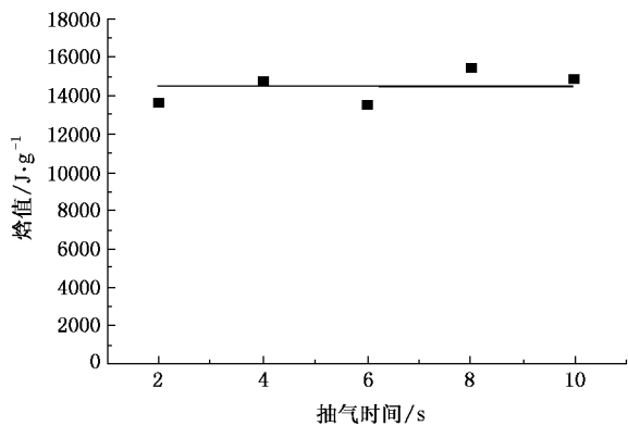
图3 不同抽气时间测量的焓值
