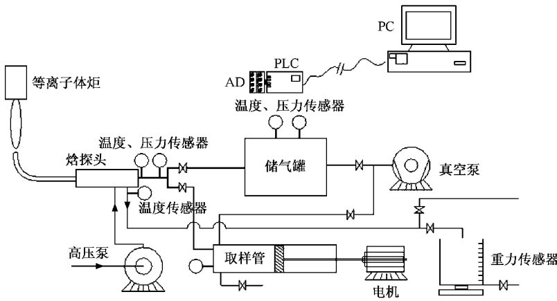
图 2 测量系统结构示意图
