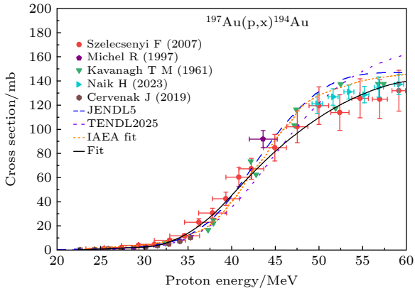
图 7 ^{197}\text{Au}(\text{p}, \text{x})^{194}\text{Au} 反应截面经修正与筛选后的实验截面数据、评价库数据及本工作评价推荐值汇总
