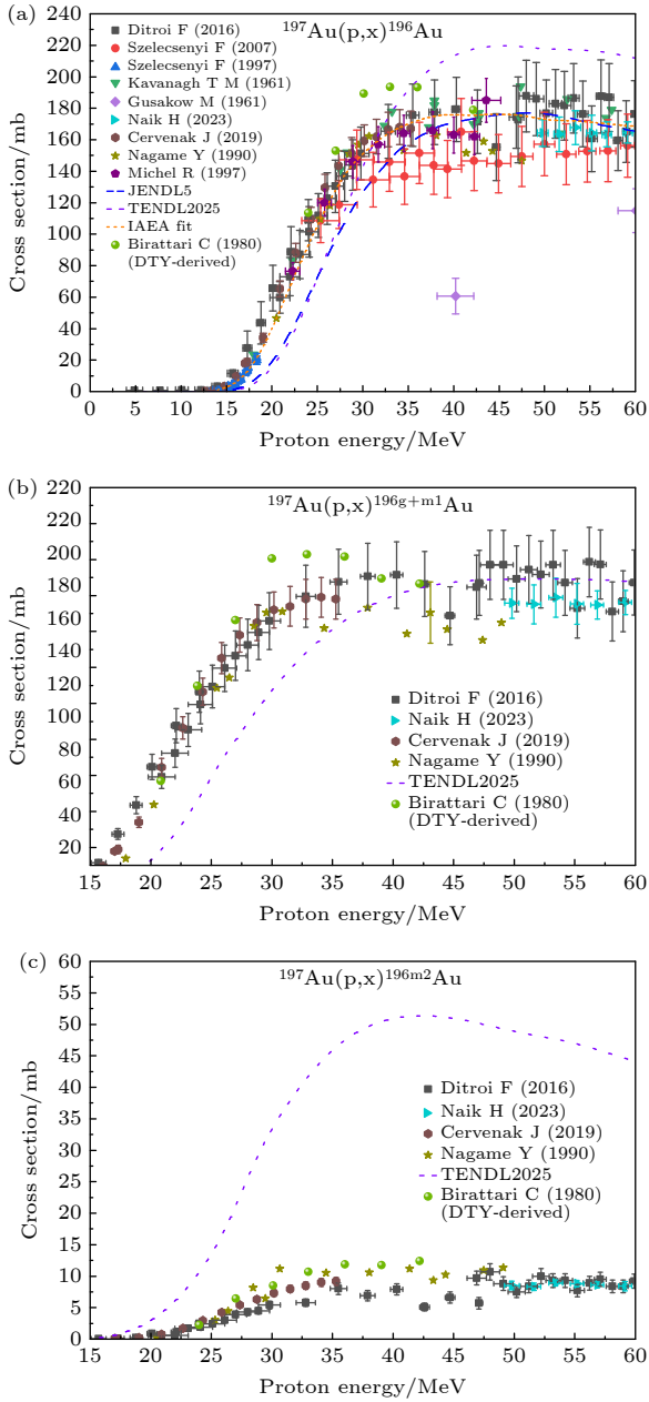
图 1 ^{197}\text{Au}(\text{p}, \text{x})^{196}\text{Au} 反应截面实验数据、评价库数据及微分厚靶产额反算截面汇总 (a)–(c) 分别为 ^{197}\text{Au}(\text{p}, \text{x})^{196}\text{Au} , ^{197}\text{Au}(\text{p}, \text{x})^{196(\text{g}+\text{m}1)\text{Au}} 和 ^{197}\text{Au}(\text{p}, \text{x})^{196\text{m}2}\text{Au} 反应道
