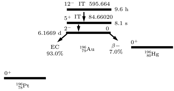
图 2 ^{196}\text{Au} 衰变纲图 (简化)
