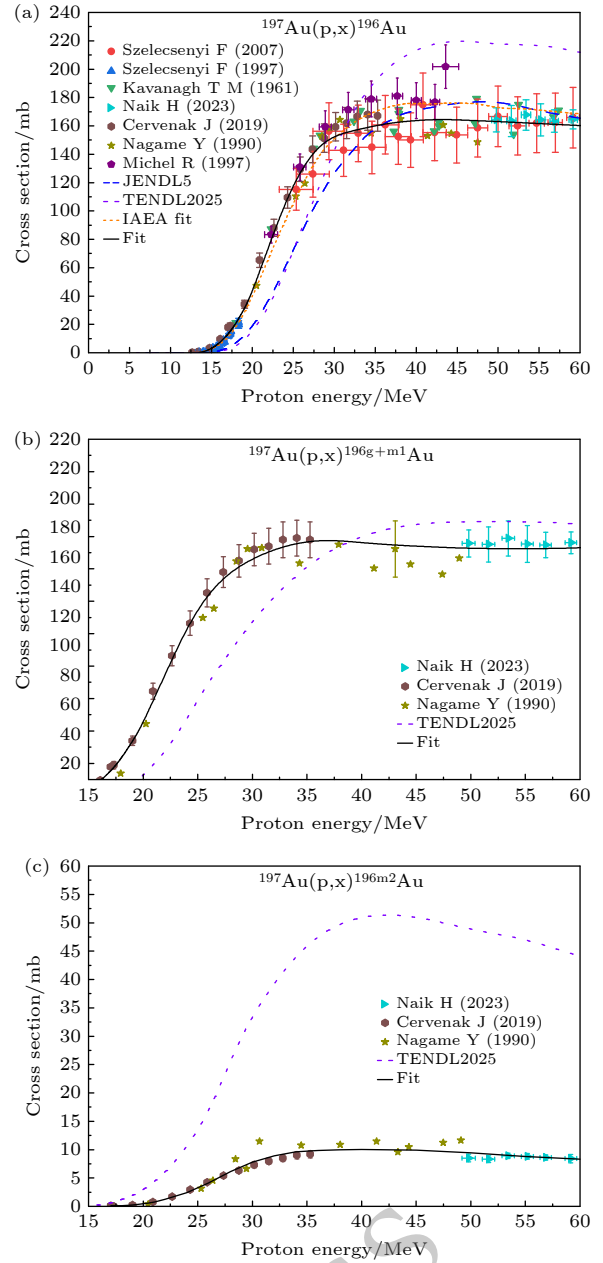
图5 ^{197}\text{Au}(\text{p}, \text{x})^{196}\text{Au} 反应截面经修正与筛选后的实验截面数据、评价库数据及本工作评价推荐值汇总 (a)–(c) 分别为 ^{197}\text{Au}(\text{p}, \text{x})^{196}\text{Au} , ^{197}\text{Au}(\text{p}, \text{x})^{196(\text{g}+\text{m}1)}\text{Au} 和 ^{197}\text{Au}(\text{p}, \text{x})^{196\text{m}2}\text{Au} 反应道
