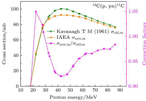
图3 Kavanagh 和 Bell (1961) [14] 使用的 12 C(p, pn) 11 C 监测截面修正因子
