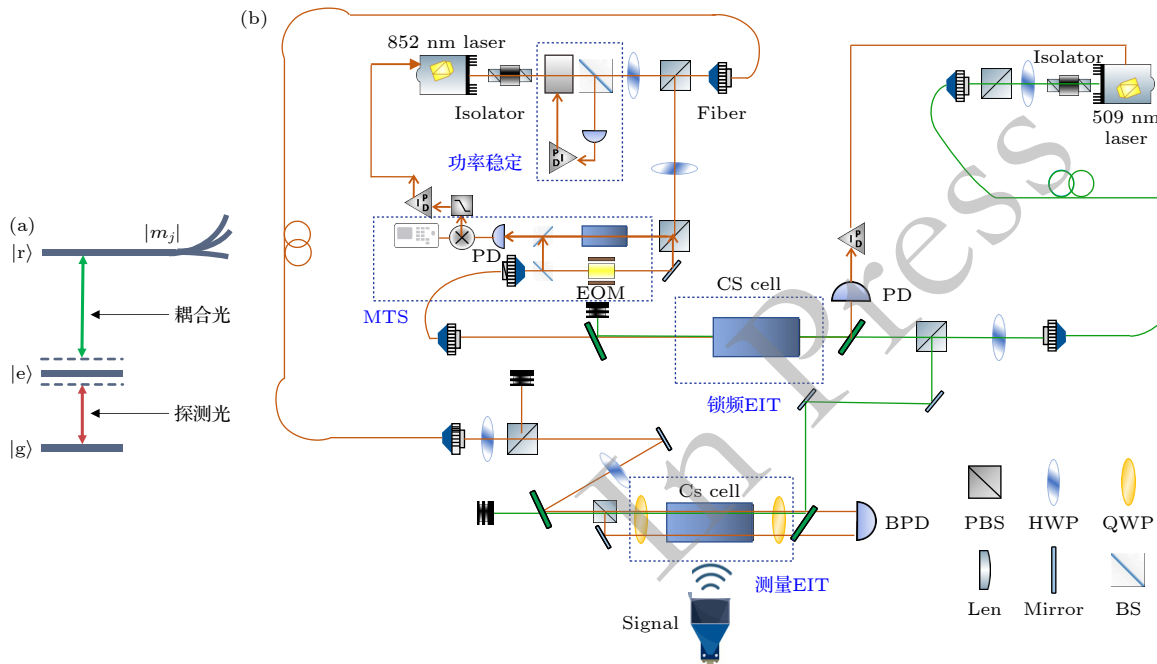
图 1 系统装置及能级图
