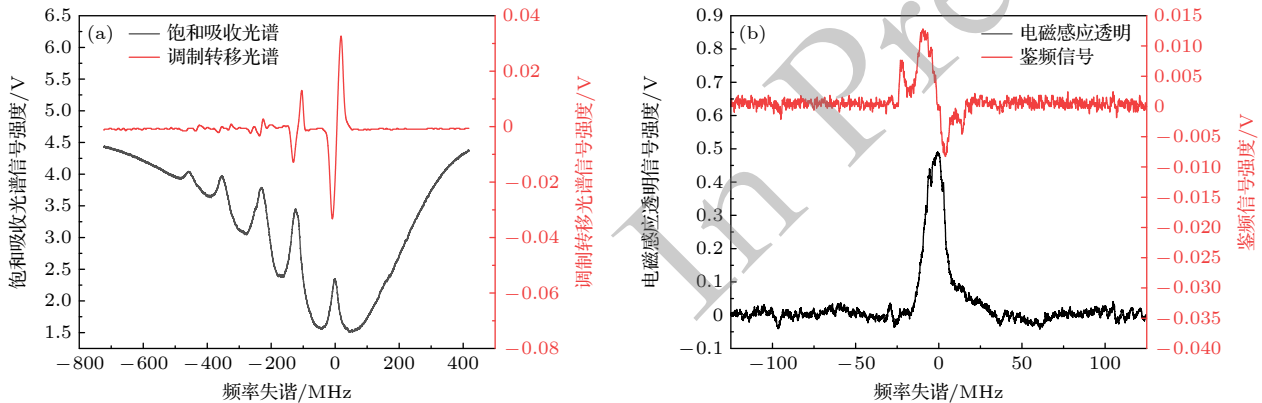
图 2 MTS-EIT 光谱信号及鉴频信号
