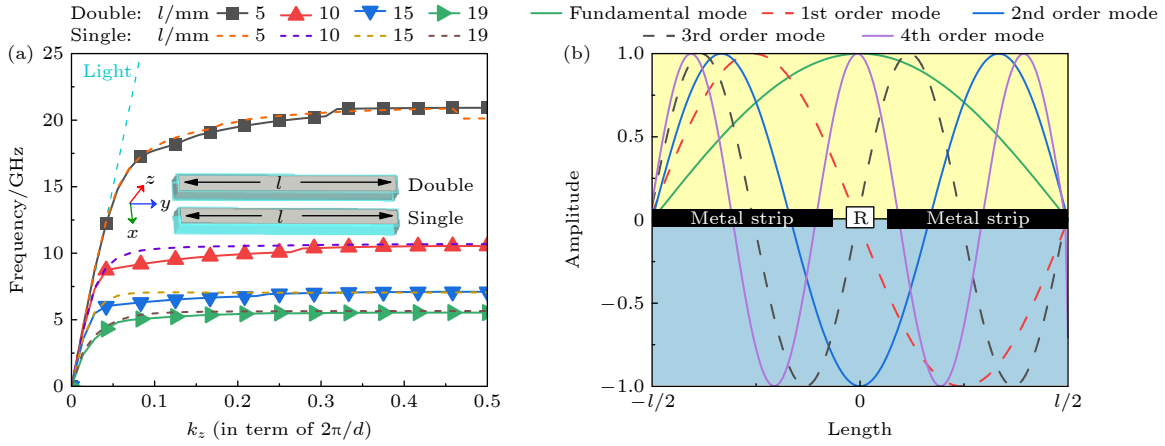
图 2 色散曲线和模式电流分析示意图 (a) 色散曲线; (b) 模式电流
