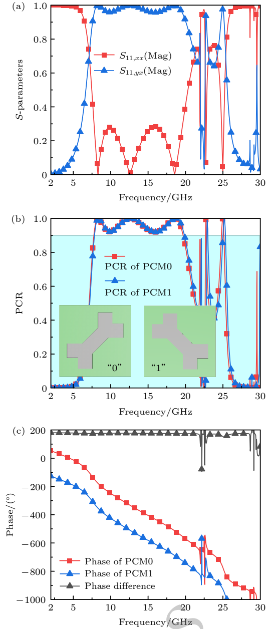
图7 极化转换超表面单元仿真结果 (a) 状态“0”单元S曲线; (b) 两种状态单元极化转换率; (c) 两种单元反射波相位
