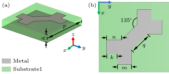
图6 极化转换超表面示意图 (a) 三维示意图; (b) 俯视图 Fig. 6. Schematic of the polarization conversion metasurface: (a) 3D view; (b) top view.
