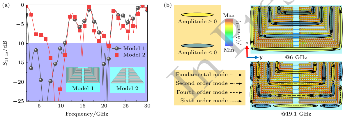
图 4 吸波器 S 曲线和 6 GHz, 19.1 GHz 表面电流 (a) S 曲线; (b) 表面电流
