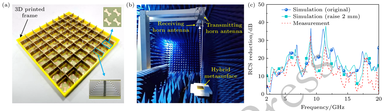
图 12 复合超表面阵列实物及测试结果 (a) 复合超表面阵列实物图; (b) 测试环境; (c) RCS 仿真与测试结果
