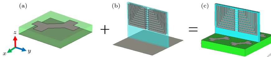
图9 复合超表面结构 (a) PCM单元; (b) SSPP吸波器单元; (c) 复合超表面单元
