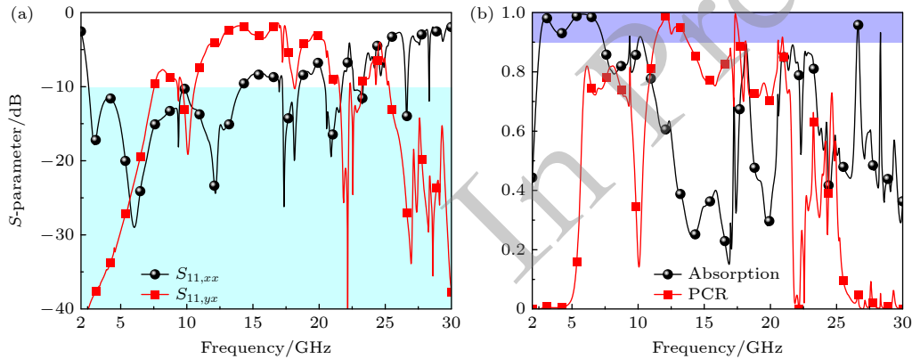
图10 复合超表面单元仿真结果 (a) S曲线; (b) 吸波率和PCR
