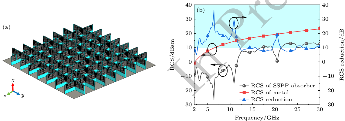
图 5 SSPP 吸波器阵列示意图及 RCS 仿真结果 (a) 阵列示意图; (b) RCS 结果
