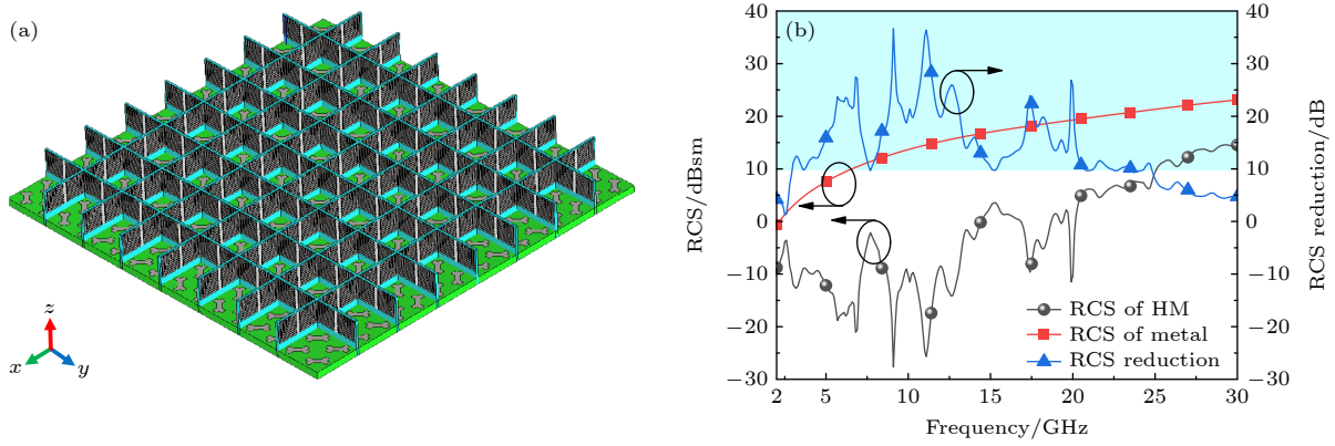
图 11 复合超表面阵列及 RCS 仿真结果 (a) 复合超表面阵列三维示意图; (b) RCS 仿真结果
