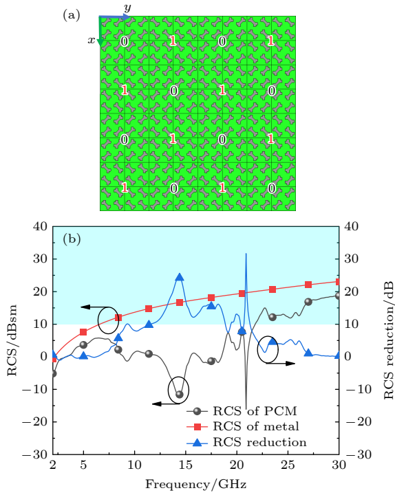
图8 棋盘PCM阵列示意图及RCS仿真结果 (a)阵列结构; (b) RCS结果
