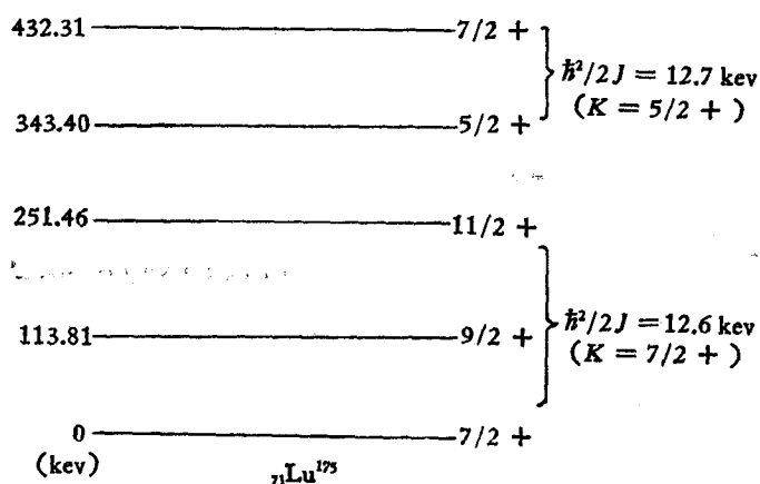
圖 4. \text{Lu}^{175} 能級圖 [9]
