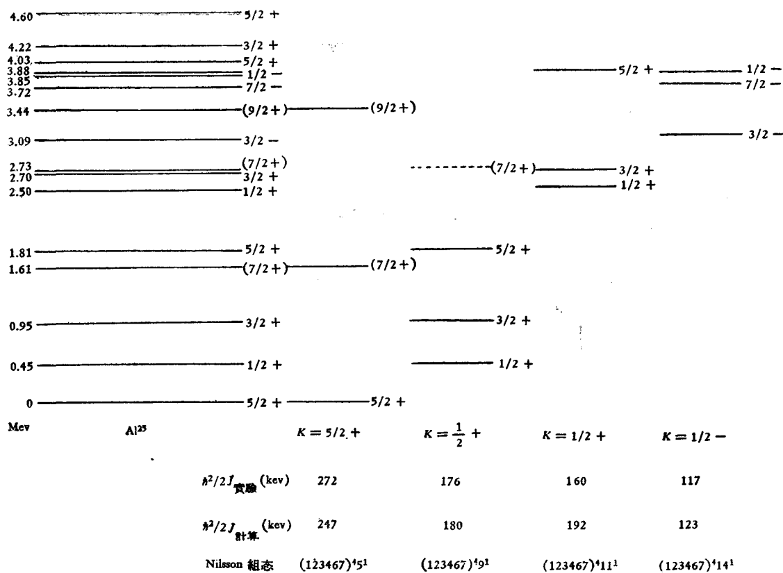
图2. Al^{25} 低激发带转动惯量(实验分析取自 D. A. Bromley 工作 [8] )
