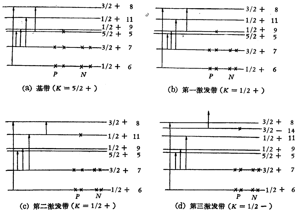
图3. Al^{25} 各激发带组态及有贡献的跃迁
