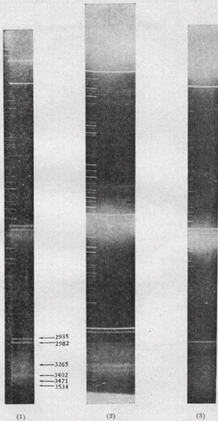
图 1. 罗谢尔土的联合散射光谱:
