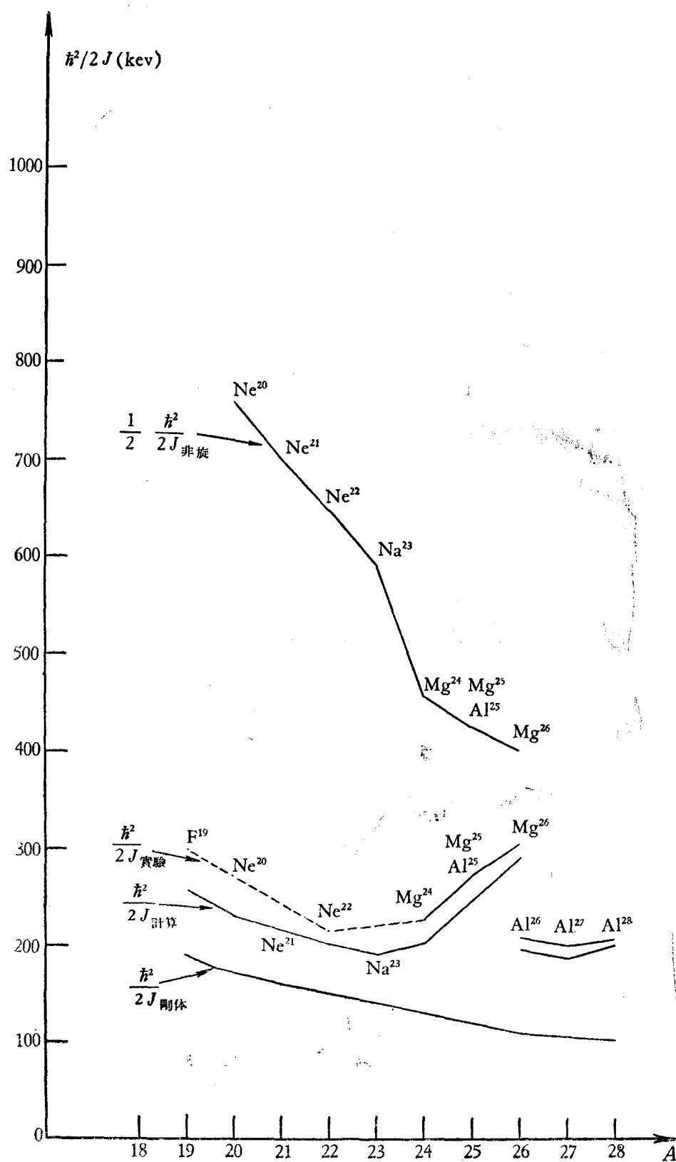
图 1. 輕核轉动区原子核轉动慣量
