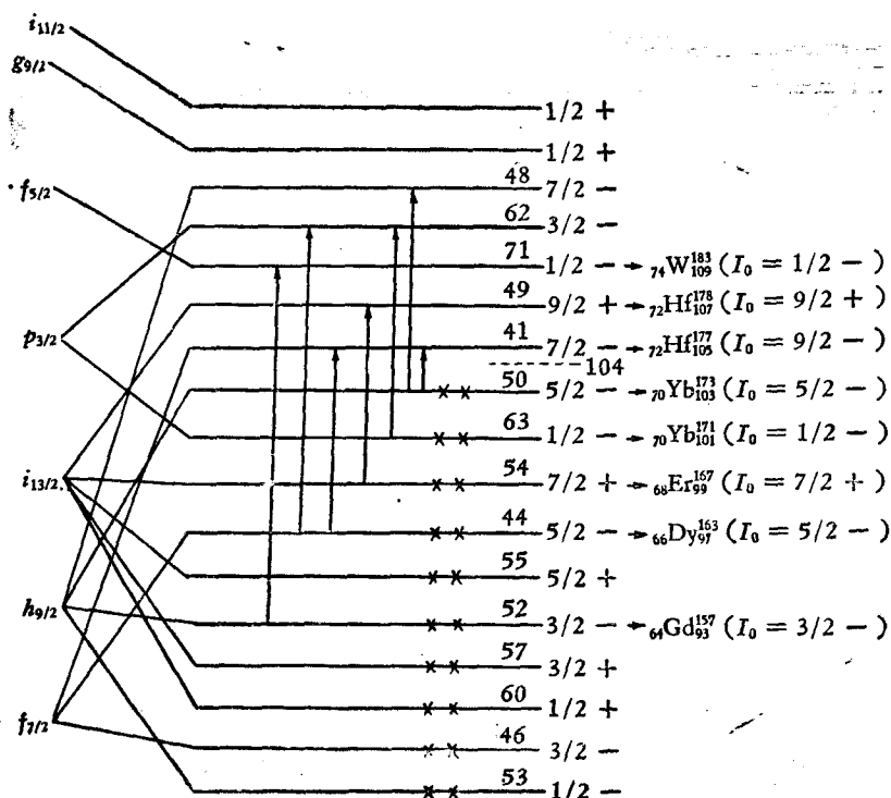
图 5(b) {}_{71}\text{Lu}_{164}^{175} 中子组态
