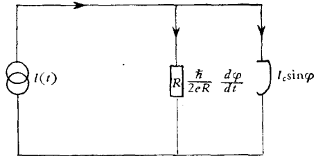
图1 电阻分路约瑟夫森结的等效电路
