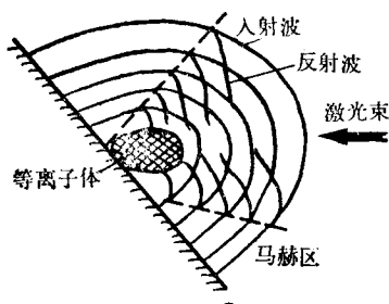
图 13 产生爆震波时椭圆形冲击波的人射反射
