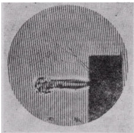
图 1 有机玻璃蒸汽羽的柱状结构
