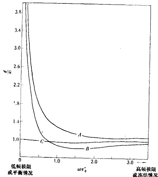
图3 相速度 a/a_f 随 \omega\tau_0^+ 的变化
