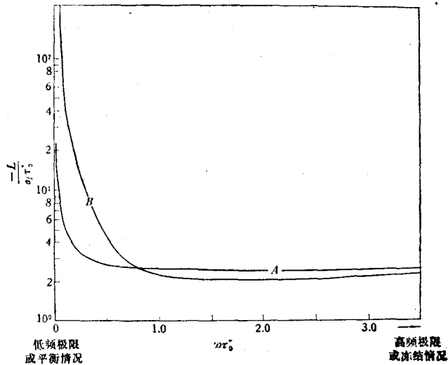
图 6 放大长度 -L/a_f \tau_0^+ 随 \omega \tau_0^+ 的变化 ( a_f/a_e=1.1 , \tau_0^+/\tau_0=1.1 ; A: Q'_p=0 , a_f^2 Q'_p \tau_0^{-1}=-1 ; B: Q'_p=0 , Q'_e \tau_0^+=-1 )
