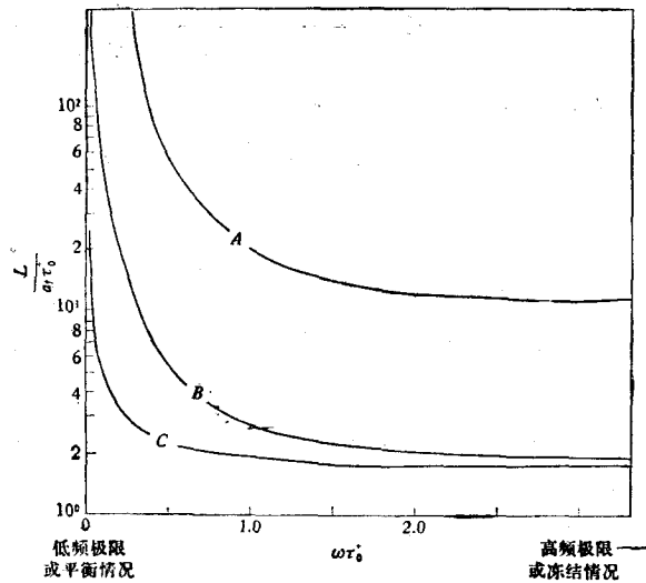
图 5 衰减长度 L/a_f \tau_0^+ 随 \omega \tau_0^+ 的变化 ( a_f/a_e=1.1 , \tau_0^+/\tau_0=1.1 ; A:指绝热情况; B 和 C 指非绝热情况; B: Q'_p=0 , Q'_e \tau_0^+=1 ; C: Q'_p=0 , a_f^2 Q'_p \tau_0^+=1 )
