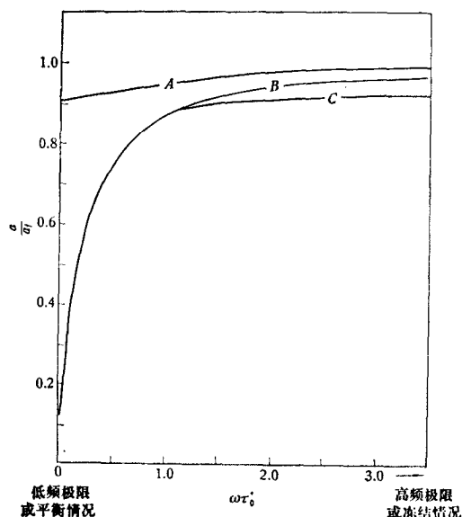
图2 相速度 a/a_f 随 \omega\tau_0^+ 的变化
