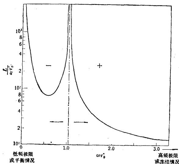
图 4 放大-衰减长度 L/a_f \tau_0^+ 随 \omega \tau_0^+ 的变化 ( a_i/a_c = 1.1 , \tau_0^+/\tau_0 = 1.1 , a_i^2 Q'_p \tau_0^+ = 1 , Q'_p \tau_0^+ = -1 ; + 为 L > 0 , 即衰减区; - 为 L < 0 , 即放大区; --- 为 (\omega \tau_0^+)^2 = 1.1 )
