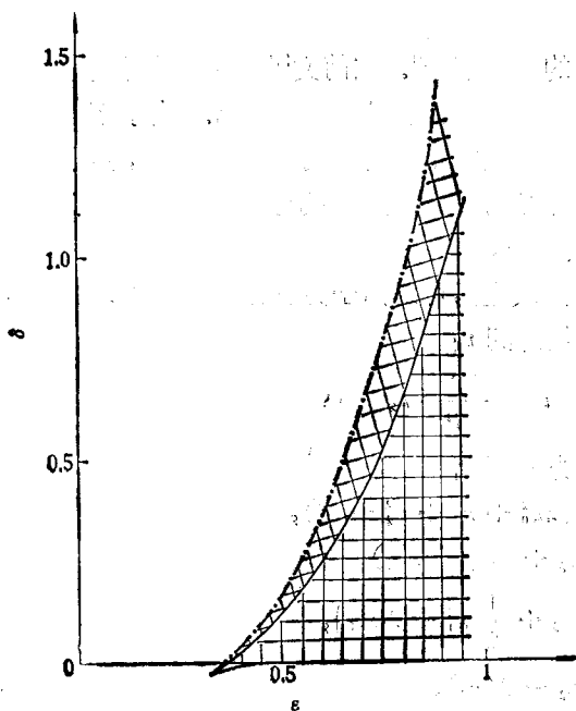
图 1 (\varepsilon, \delta) 平面上栅为定态解和斜线为周期解的稳定区
