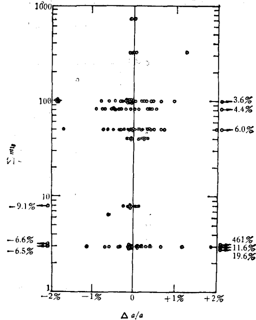
图2 各组方程组正矩阵 M 的第 1 行元素绝对值之和与 \Delta a/a 的关系数据点分布无规律;图外的数据用箭号表示,箭号下数字为横坐标值
