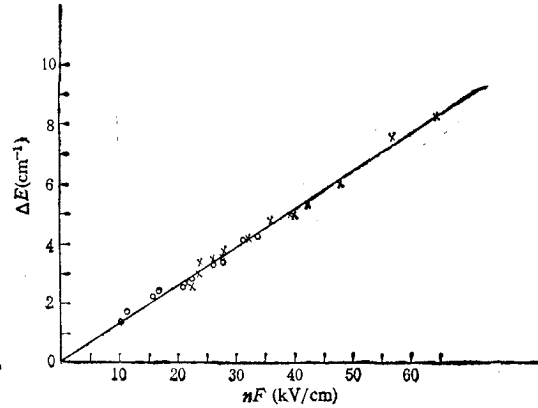
图 4 Sr 和 Ca 原子 Stark 能级分裂与外场强 nF 关系 × 为 Sr 原子测量值; ○ 为 Ca 原子测量值; 直线为 \Delta E = 3nF(\text{au})
