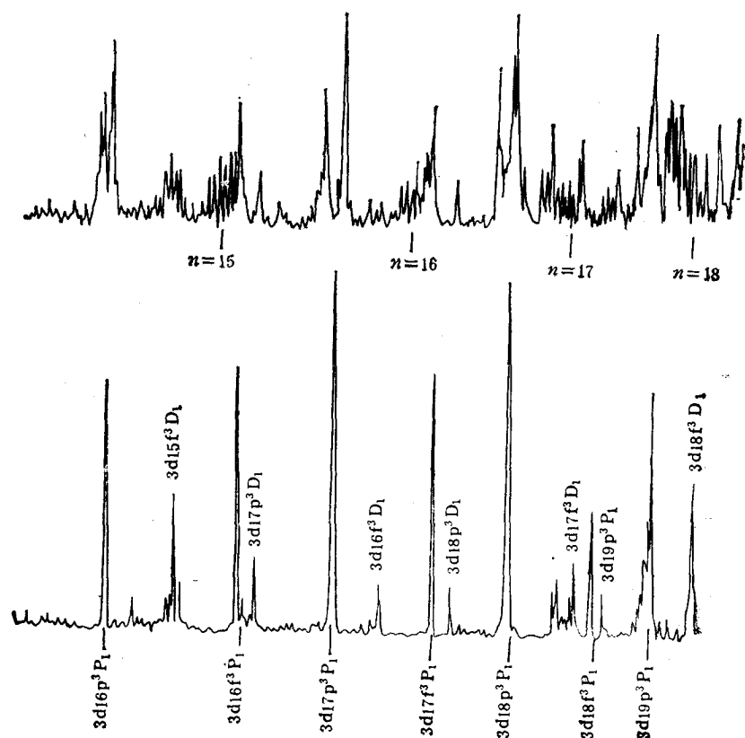
图 2 Ca 原子 3dnl 自电离态的 Stark 光谱
