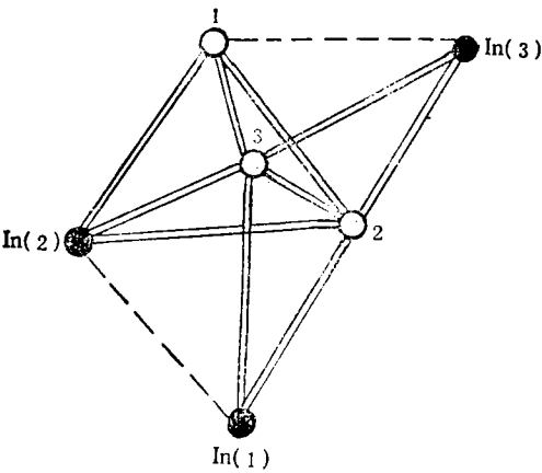
图 4 \text{In}_3\text{P}_3^+ 的构型
