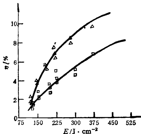
图 4 DCCTA 透射光栅的 \eta 与 E 之间的关系曲线 \square 为未烘烤; \triangle 为 80^\circ\text{C} , 烘烤 30min
