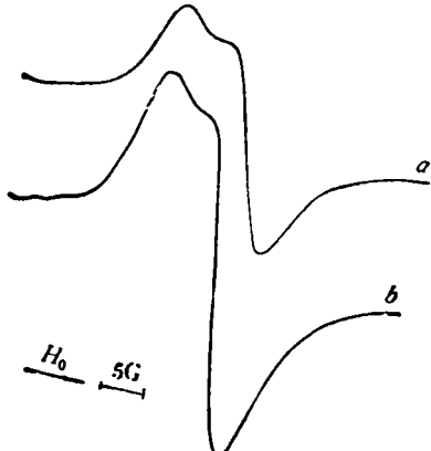
图 3 DCCTA 室温下的 EPR 谱
