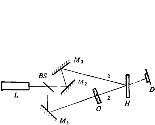
图 1 记录 DCCTA 透光光栅的实验原理图
