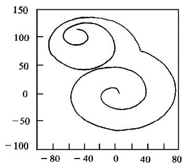
图6 双螺旋波形
