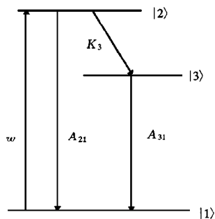
图 7 Rb 原子的基态和第一激发态能级简图
