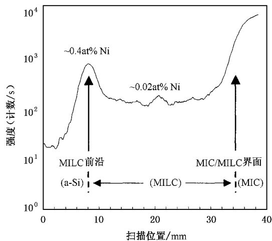
图 2 使用二次离子谱所得到的 Ni 在 MIC, MILC 以及 a-Si 区间的一维分布图
