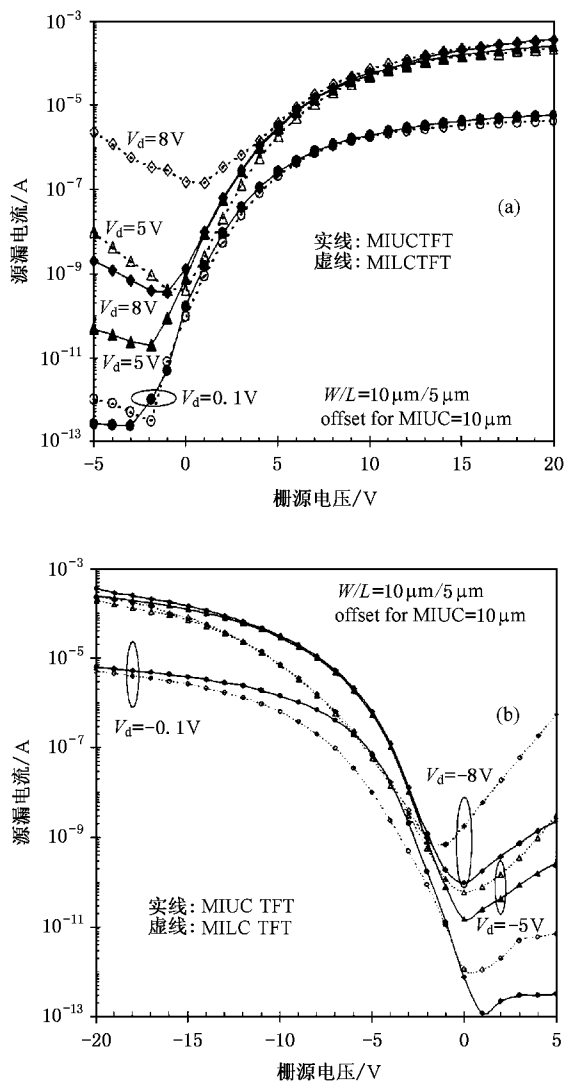
图 4 各种不同源漏电压 ( V_{ds} ) 下的源漏电流 ( I_{ds} ) 和栅源电压 ( V_{gs} ) 对应曲线((a)为 n 沟器件 (b)为 p 沟器件)
