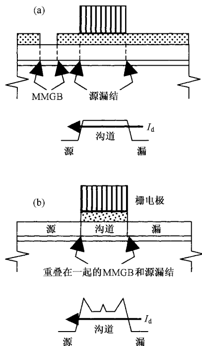
图 3 器件沟道的剖面示意图((a)为“000” MILC TFT,MMGB 已被移出结区.(b)为“111”MILC TFT,MMGB 与结区重叠)
