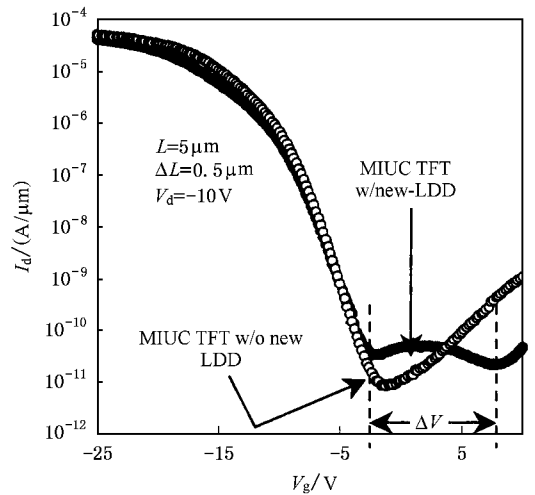
图9 具有新型栅控 LDD 结构和没有 LDD 结构 MIUC-TFT 的转移特性曲线
