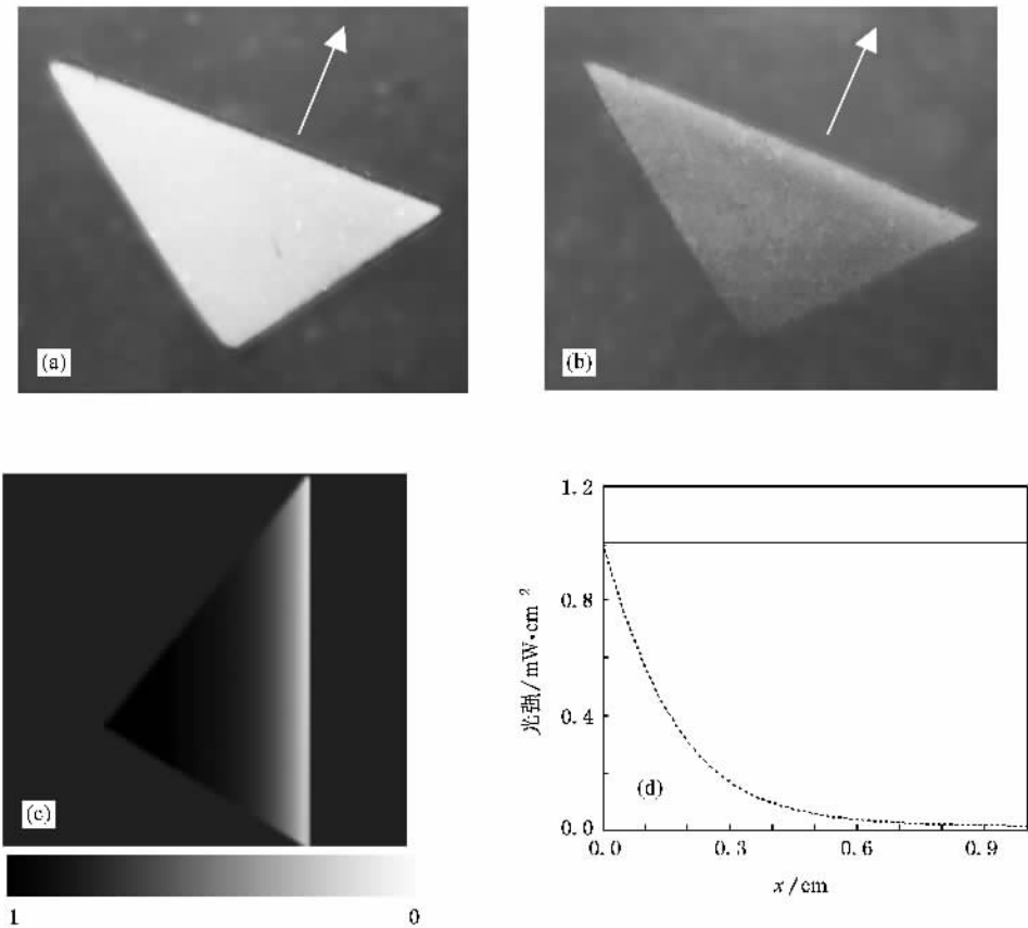
图1 当输入图像的光强为均匀分布时的输出图像 (a)实验输入图像 (b)实验得到的输出图像 (c)当物体运动速度 v = 0.1\text{ cm/s} 在 t = 10\text{ s} 时数值模拟得到的灰度图像 (d)输入图像(实线)和输出图像(虚线)的蓝光光强分布
