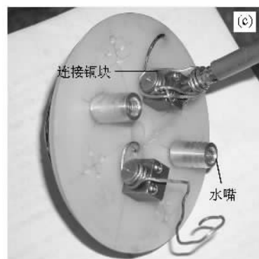
图2 制作完成的 Ioffe 线圈照片 (a)第一组 Ioffe 线圈 (b)第二组 Ioffe 线圈 (c)第一组 Ioffe 线圈的侧视图
