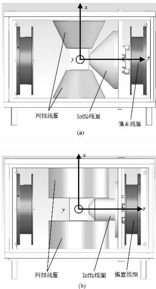
图1 四极线圈和 Ioffe 线圈的组合示意图 (a)第一组线圈, (b)第二组线圈
