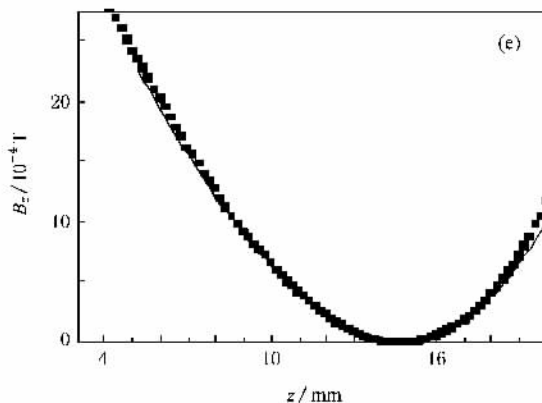
图3 四级线圈电流为 25.1 A 时,第一组线圈组合的四极磁阱向 QUIC 磁阱的转变过程 (a)(c)(e)为数值模拟结果(曲线)与实验结果(数据点)的对比 (b)(d)(f)为与(a)(c)(e)相应的原子吸收成像照片. Ioffe 线圈的电流从上而下分别为 0, 16.6 和 18 A. 相对于 (a) 图 (c) 和 (e) 的成像系统分别移动了约 8 和 11 mm
