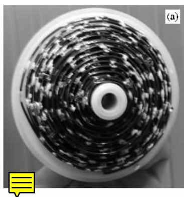
图2 制作完成的 Ioffe 线圈照片 (a)第一组 Ioffe 线圈 (b)第二组 Ioffe 线圈 (c)第一组 Ioffe 线圈的侧视图
