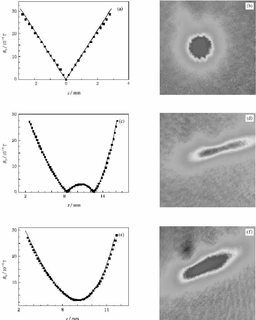
图4 四极线圈电流为 25.1 A 时, 第二组线圈组合的四极磁阱向 QUIC 磁阱的转变过程 (a)(c)(e) 为数值模拟结果(曲线)与实验结果(数据点)的对比 (b)(d)(f) 为与(a)(c)(e) 相应的原子吸收成像照片. Ioffe 线圈的电流从上而下分别为 0.33 和 35 A. 相对于(a)图 (c) 和 (e) 的成像系统分别移动了约 7 和 9 mm
