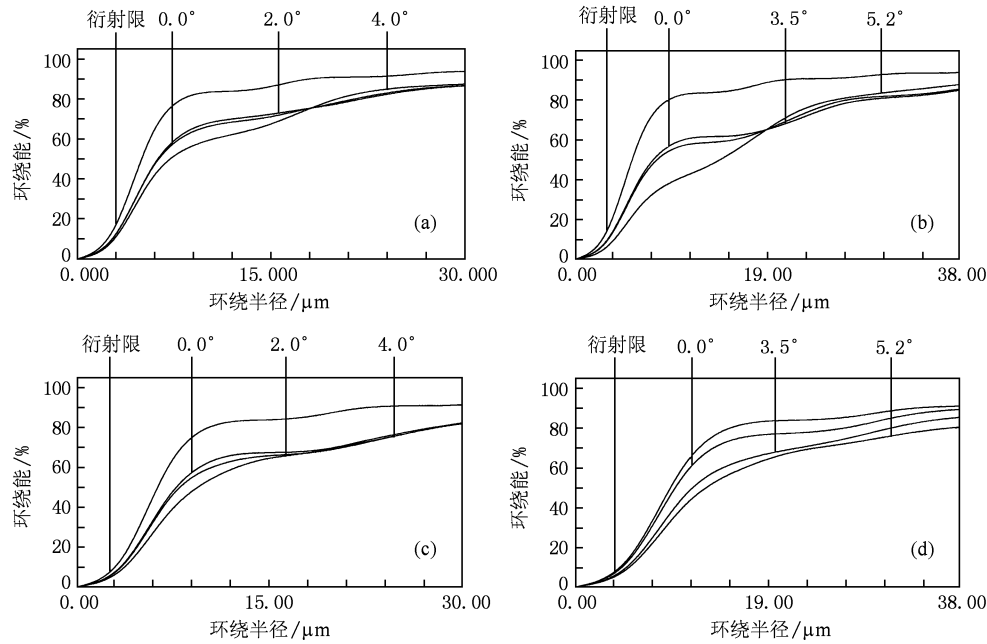
图 7 光学系统在各波长处的环绕能量曲线图 (a) 3.7 \mu\text{m} , (b) 4.8 \mu\text{m} , (c) 8 \mu\text{m} , (d) 12 \mu\text{m}
