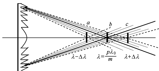
图 1 谐衍射元件的色散
