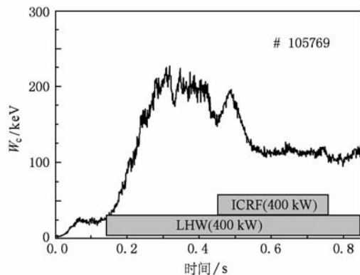
图10 #105769 逃逸电子的逃逸阈值
