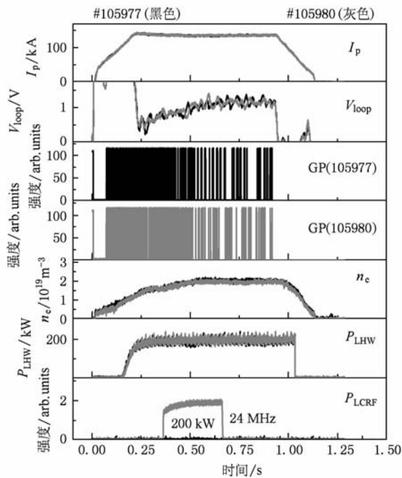
图5 #105977 和#105980 放电波形图
