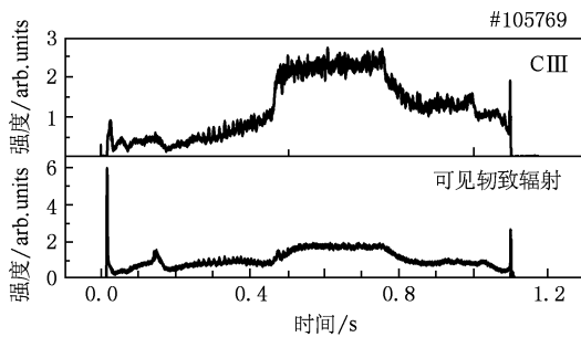
图9 #105769 放电过程中辐射波形图
