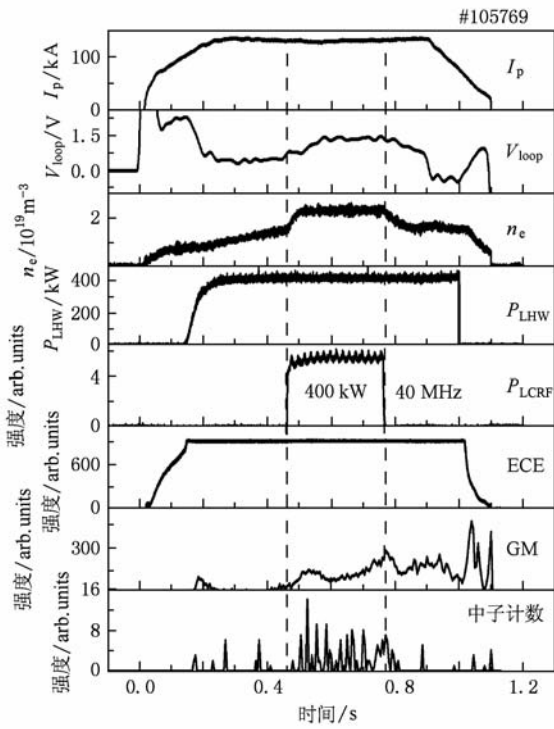
图7 #105769 放电波形图
