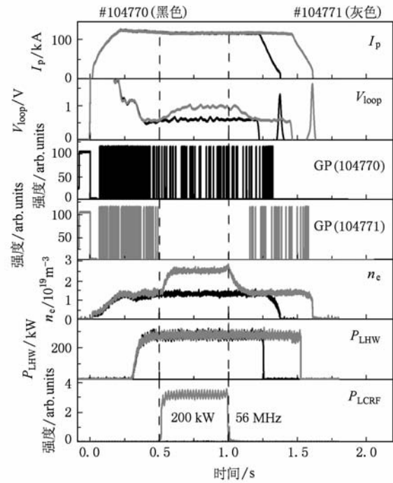
图 1 #104770 和 #104771 放电波形图
