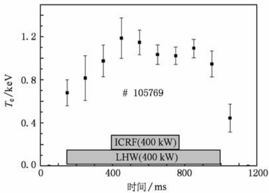
图8 #105769 软 X 射线能谱测量得出的电子温度
