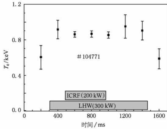
图3 #104771 软 X 射线能谱测量得出的电子温度
