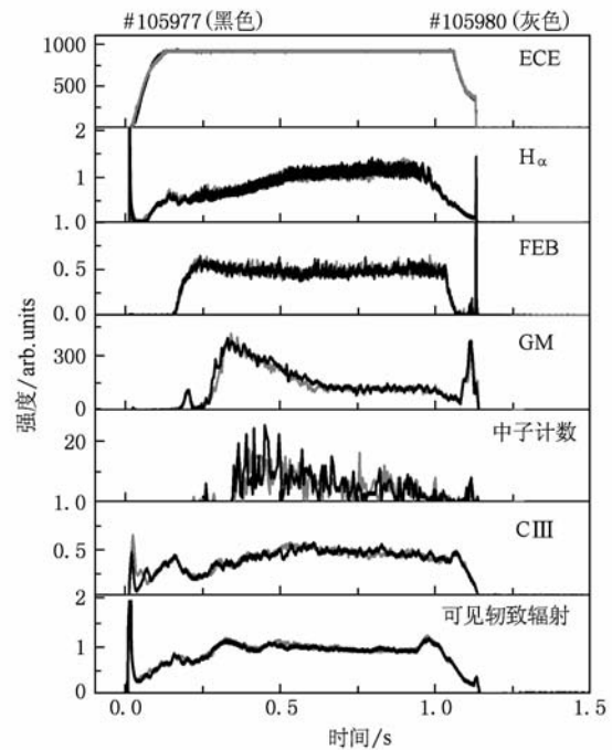
图6 #105977 和#105980 放电等离子体辐射参数图
