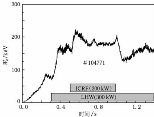
图4 #104771 逃逸电子的逃逸阈值
