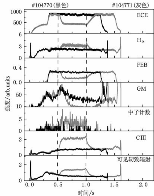
图 2 #104770 和 #104771 放电等离子体辐射参数图 ECE 为电子回旋辐射强度, H\alpha 为 H\alpha 线辐射强度, FEB 为快电子韧致辐射强度, GM 为 \gamma -射线辐射强度, CIII 为碳杂质辐射强度
