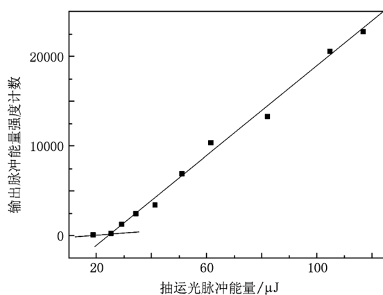
图 7 激光输出特性曲线
