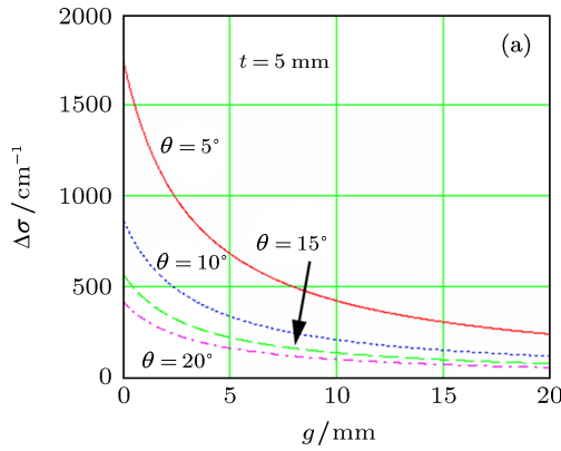
图 4 SZBIS 光谱分辨率 \Delta\sigma_{\text{SZBIS}} 与 PDWP 分束器参数间的关系 (方解石, \lambda = 0.6328 \mu\text{m} )
