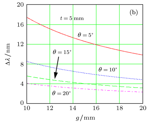
图 5 SZBIS 光谱分辨率 \Delta\lambda_{\text{SZBIS}} 与 PDWP 分束器参数间的关系 (方解石, \lambda = 0.6328 \mu\text{m} )
