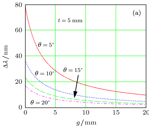
图 5 SZBIS 光谱分辨率 \Delta\lambda_{\text{SZBIS}} 与 PDWP 分束器参数间的关系 (方解石, \lambda = 0.6328 \mu\text{m} )
