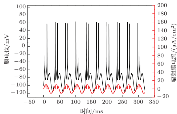
图4 神经元膜电位 ( v ) 和电磁辐射产生的辐射膜电流 ( \Delta I ) 的时间序列(其中电磁辐射强度 S = 50 , 电磁辐射频率 f = 1800 \text{ MHz} , 刺激电流 I_{\text{stim}} = 5 )
