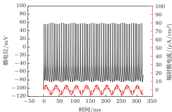
图5 神经元膜电位 ( v ) 和电磁辐射产生的辐射膜电流 ( \Delta I ) 的时间序列(其中电磁辐射强度 S = 50 , 电磁辐射频率 f = 1800 \text{ MHz} , 刺激电流 I_{\text{stim}} = 20 )
