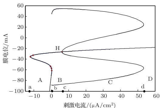
图3 电磁辐射强度 S 为零时神经膜电位 v 关于刺激电流 I_{\text{stim}} 的分岔图(点 a, b, c, d 将横坐标轴分为 4 个区间: A 表示稳定的平衡态; B 表示含有一个极限环的单稳态; C 表示双稳态; D 表示静息状态)
