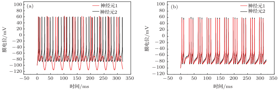
图7 神经元1(受到 S = 50 , f = 1800 MHz 的磁辐射)的簇放电模式对神经元2(无电磁辐射影响)放电行为的影响 (a) 耦合强度 D = 0 ; (b) 耦合强度 D = 1
