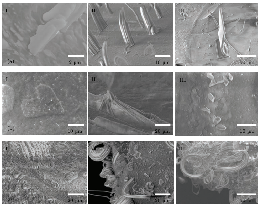
图2 不同浓度的钠盐溶液在多孔硅胶颗粒表面的结晶形态 (a) NaCl 溶液浓度分别为(I) 0.5 mol/kg, (II) 1 mol/kg, (III) 4 mol/kg, 多孔硅胶颗粒的平均孔径为9 nm; (b) \text{Na}_2\text{SO}_4 溶液浓度分别为(I) 1 mol/kg, (II) 1.5 mol/kg, (III) 2 mol/kg, 多孔硅胶颗粒的平均孔径为4 nm; (c) \text{NaNO}_3 溶液浓度分别为(I) 1 mol/kg, (II) 3 mol/kg, (III) 5 mol/kg, 多孔硅胶颗粒的平均孔径为15 nm
