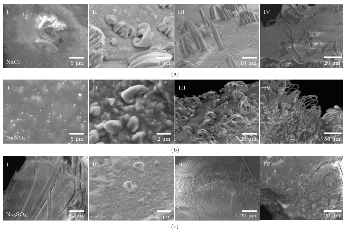
图 1 \text{NaCl} (a), \text{NaNO}_3 (b), \text{Na}_2\text{SO}_4 (c) 水溶液在不同孔径多孔硅胶颗粒表面上形成的结晶形态; 多孔硅胶颗粒的平均孔径分别为 (I) 2 nm, (II) 4 nm, (III) 9 nm, (IV) 15 nm; 三种盐溶液的浓度分别为 \text{NaCl} , 1 mol/kg; \text{NaNO}_3 , 3 mol/kg; \text{Na}_2\text{SO}_4 , 1 mol/kg
