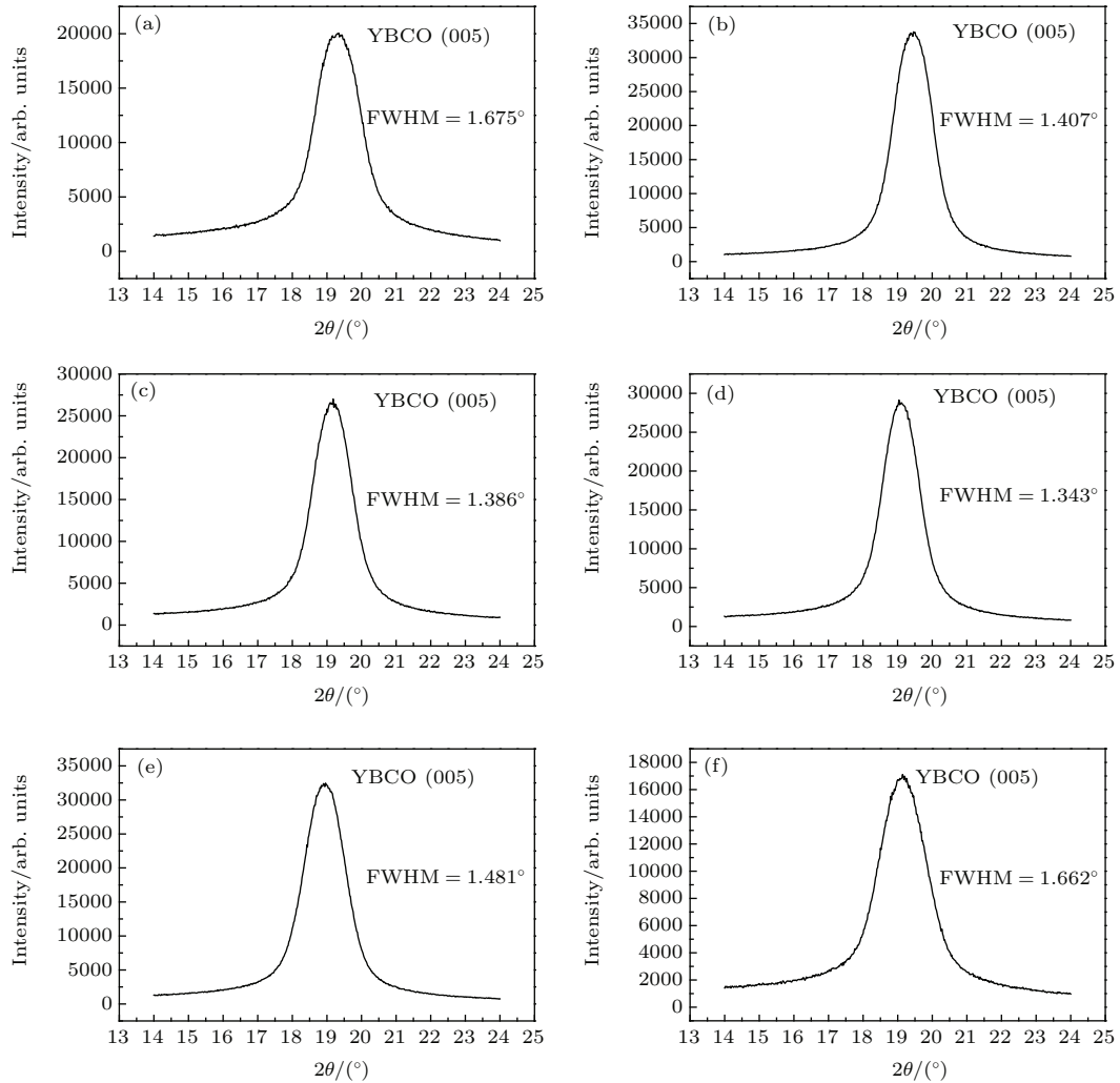
图 5 在不同溅射时间沉积的 \text{CeO}_2 插层膜上所制备的 YBCO 厚膜的 XRD(005) \omega 扫描 (a) 2 min; (b) 5 min; (c) 10 min; (d) 15 min; (e) 20 min; (f) 25 min
