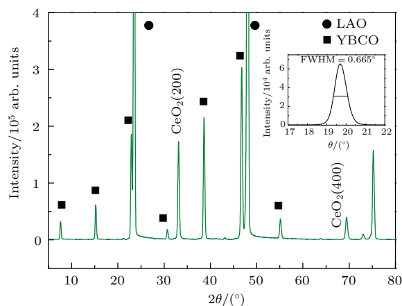
图1 制备的 LAO/CeO 2 (RF-sputtering)/BTO-YBCO(TFA-MOD) 薄膜的 XRD \theta -2 \theta 扫描谱和 (005) \omega 扫描图
