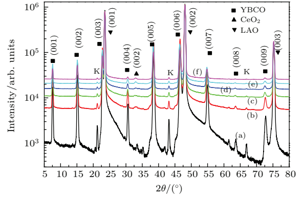
图 4 (网刊彩色) 在不同溅射时间沉积的 \text{CeO}_2 插层膜上制备的 YBCO 厚膜的 XRD \theta - 2\theta 扫描谱 (a) 2 min; (b) 5 min; (c) 10 min; (d) 15 min; (e) 20 min; (f) 25 min
