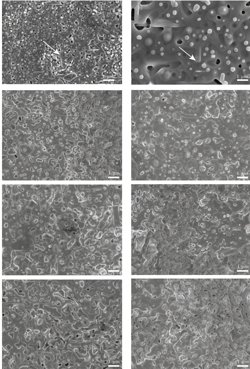
图 3 在不同溅射时间沉积的 \text{CeO}_2 插层膜上制备的 YBCO 厚膜的 SEM 照片 (a) 2 min; (b) 5 min; (c) 10 min; (d) 15 min; (e) 20 min; (f) 25 min; (g) 25 min; (h) 25 min
