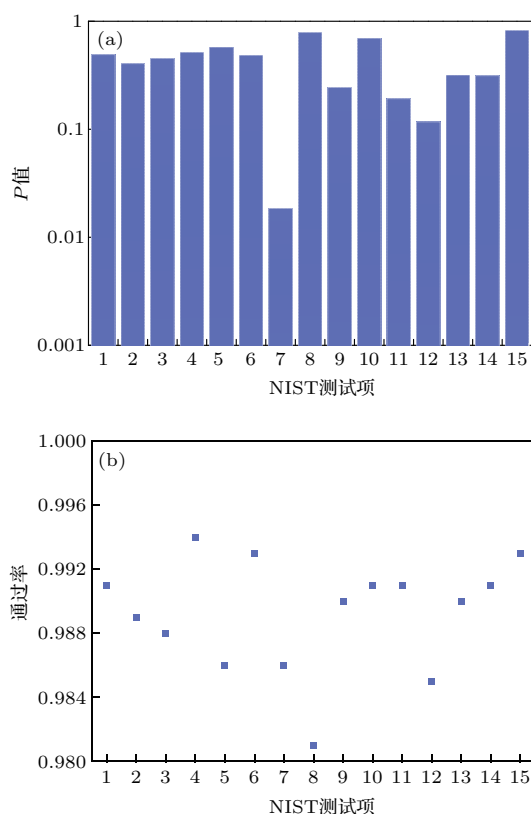
图6 NIST 测试结果 (a) 各测试项的 P 值; (b) 各测试项的通过率
