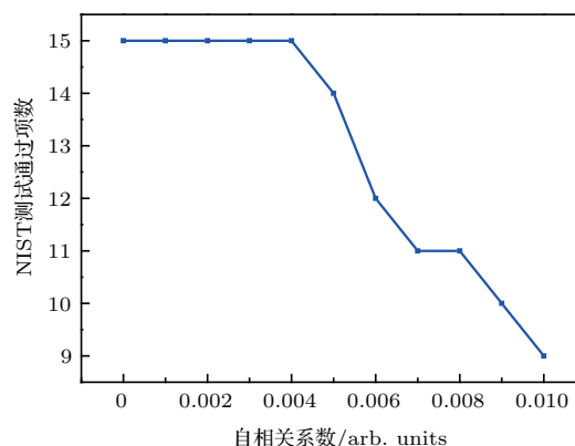
图7 不同的混沌脉冲自相关系数下, 通过 NIST 测试的项数变化情况
