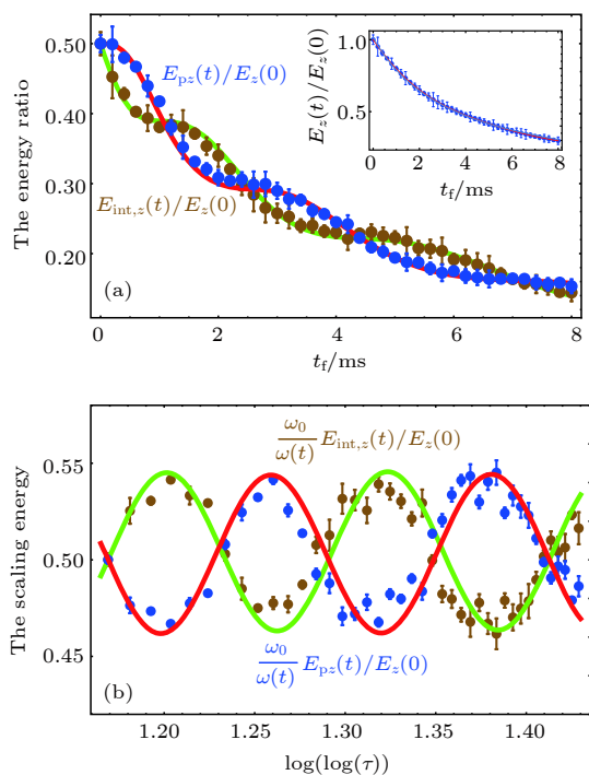
图 7 超级 Efimovian 膨胀过程中的内能和势能在时间 (a) 及其双对数标度 (b) 下的变化示意图 [42]
