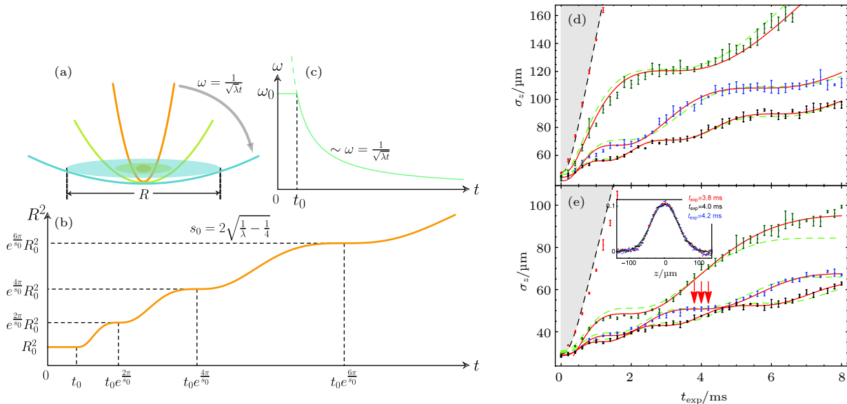
图 4 Efimovian 膨胀动力学示意图 (a), (b) 原子气体所处谐振子阱频率的变化过程; (c) Efimovian 膨胀动力学的理论预测; (d), (e) 分别代表无相互作用费米气体和强相互作用费米气体的 Efimovian 膨胀动力学的实验观测结果 [16]
