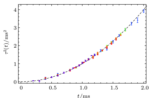
图 2 么正费米气体和无相互作用费米气体的标度不变展开动力学 [34]
