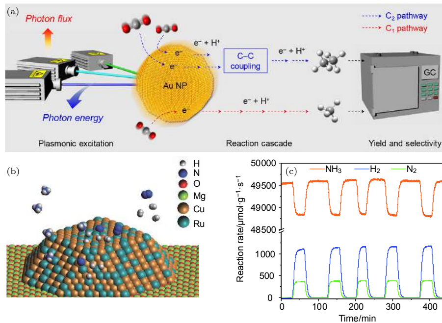
图 8 (a) Au NPs 等离子体诱导的光催化 CO 2 转化成烃的反应系统示意图, 其中通过 GC 监测反应产物与反应速率 [59] ; (b) 铜钌合金天线反应器 (Cu-Ru-AR) 的结构示意图, 其由 Cu-Ru 表面合金组成; (c) 利用 GC 监测获得的 Cu-Ru-AR 的光催化速率 (9.6 W/cm 2 ) [5]
