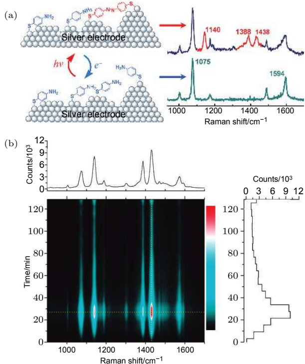
图 2 (a) 通过 SERS 光谱检测的 Ag 基底上 PATP 分子到 DMAB 分子的转变 [31] ; (b) 在 Ag 纳米颗粒上 PATP 分子反应生成 DMAB 分子的时间依赖 SERS 光谱 [32] Fig. 2. (a) Conversion of PATP molecules to DMAB molecules on Ag substrate and the SERS spectroscopy [31] ; (b) time-dependent SERS spectroscopy of DMAB molecules generated by PATP molecule reaction on Ag nanoparticles [32] .
