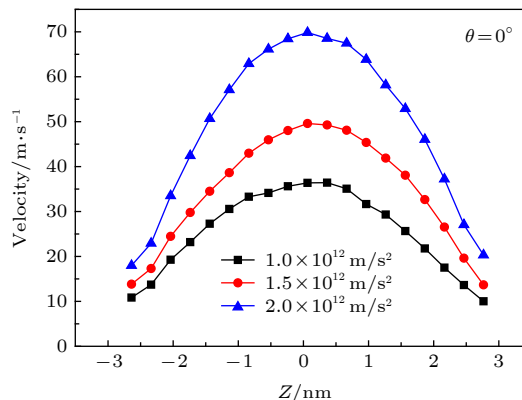
图 2 模型手性角度为 0^\circ 时水分子的速度分布
