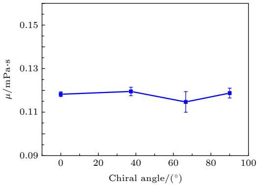
图 5 不同手性的模拟系统在不同加速度条件下的水分子黏度系数方差分布图
