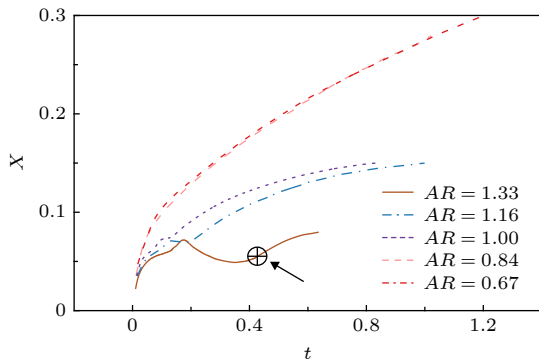
图 11 自由表面下涡环的最大涡量横向位置随时间变化 ( Fr = 112.5 , We = 145 , Re = 1740 , V_i = 6 m/s)
