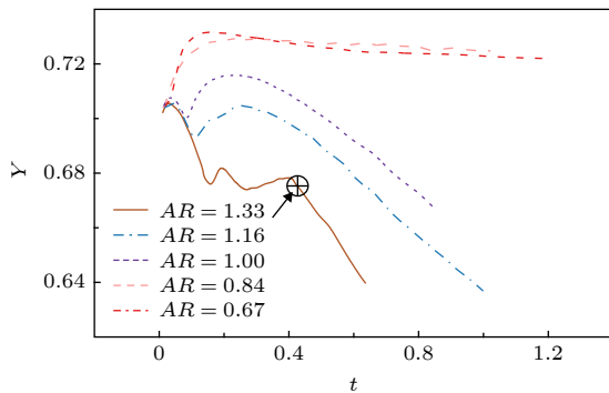
图 12 自由表面下涡环的最大涡量垂向位置随时间变化 ( Fr = 112.5 , We = 145 , Re = 1740 , V_i = 6 m/s)
