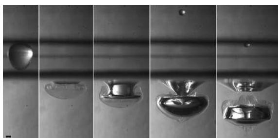
图 3 实验摄得自由液面随时间运动过程 [31]
