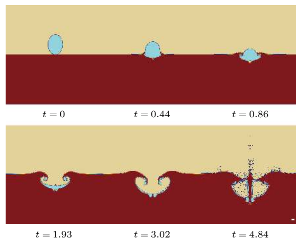
图 4 数值模拟自由液面随时间运动过程
