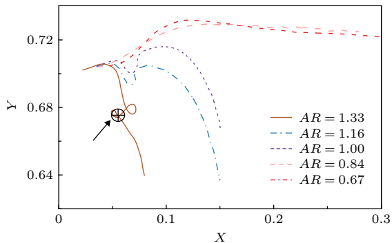
图 10 自由表面下涡环的最大涡量位置随时间变化 ( Fr = 112.5 , We = 145 , Re = 1740 , V_i = 6 \text{ m/s} )
