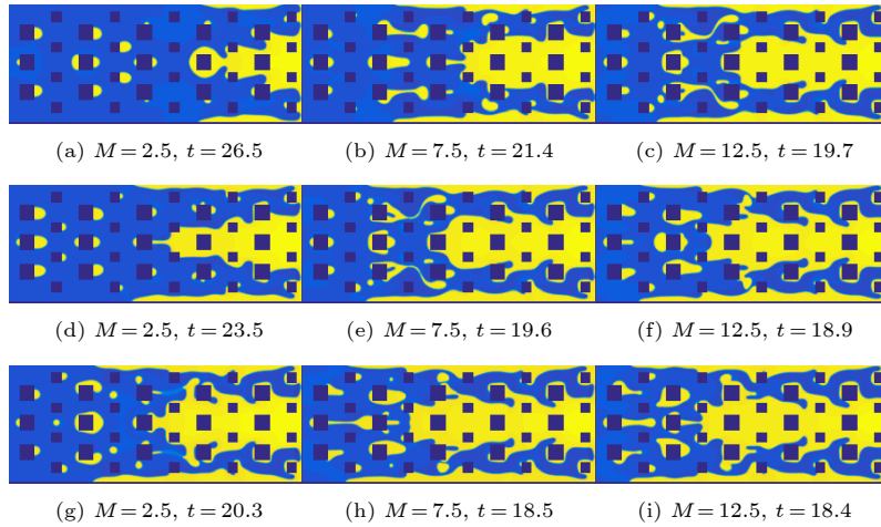
图 11 不同的动力黏性比 M 下, 被驱替液为剪切变稀、牛顿与剪切变稠流体时得到的指进形态图 (a)—(c) n = 0.7 ; (d)—(f) n = 1.0 ; (g)—(i) n = 1.3
