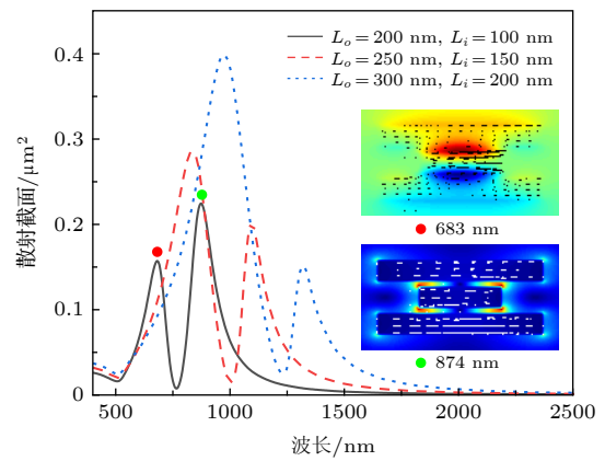
图 5 金纳米棒三聚体的散射谱随三棒尺寸变化的关系, 插图 为在指定散射共振峰位处的纳米结构截面电磁场和电 流密度矢量分布
